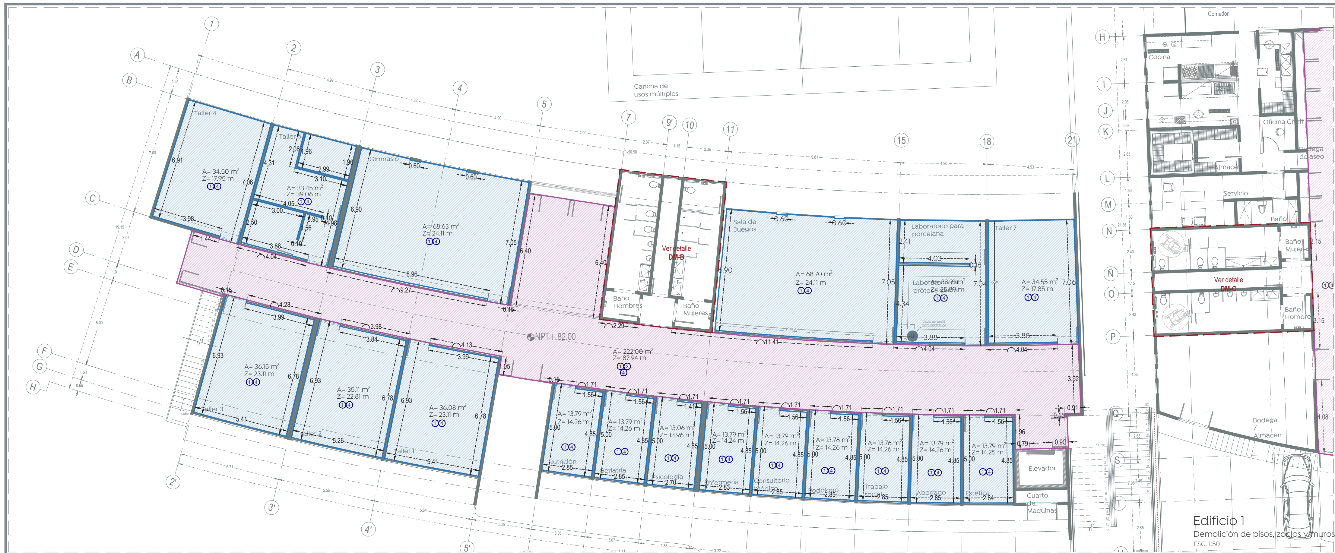
DM-C Demolición de piso, azulejo y zoclos ESC. 1:75
