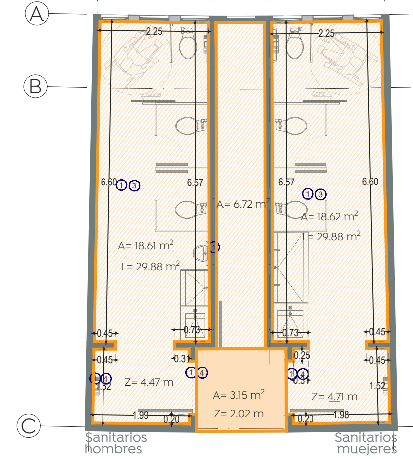
DM-B Demolición de piso, azulejo y zoclos ESC. 1:75
