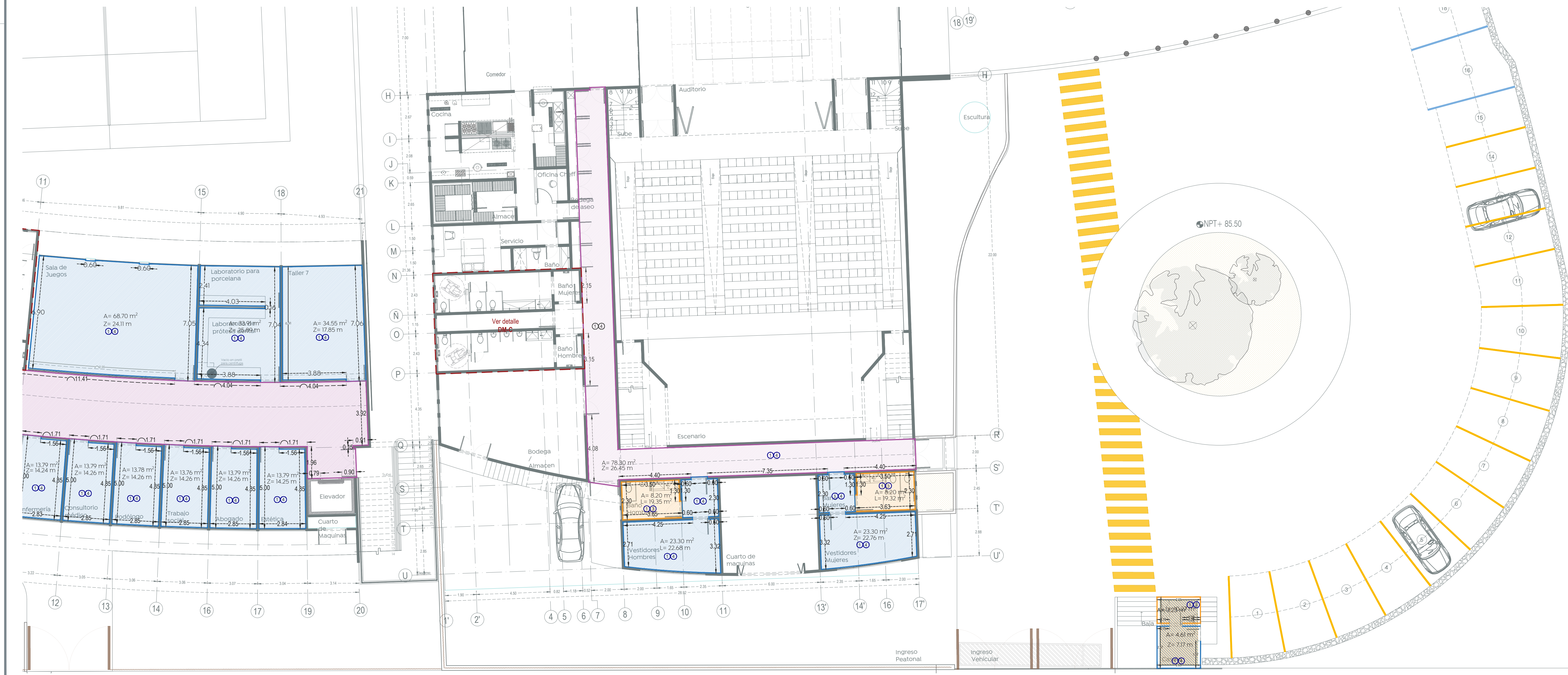
DM-B Demolición de piso, azulejo y zoclos ESC. 1:75
