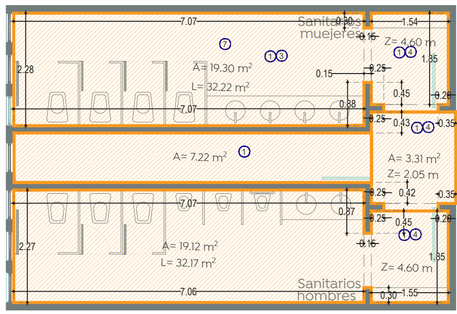
DM-C Demolición de piso, azulejo y zoclos ESC. 1:75
