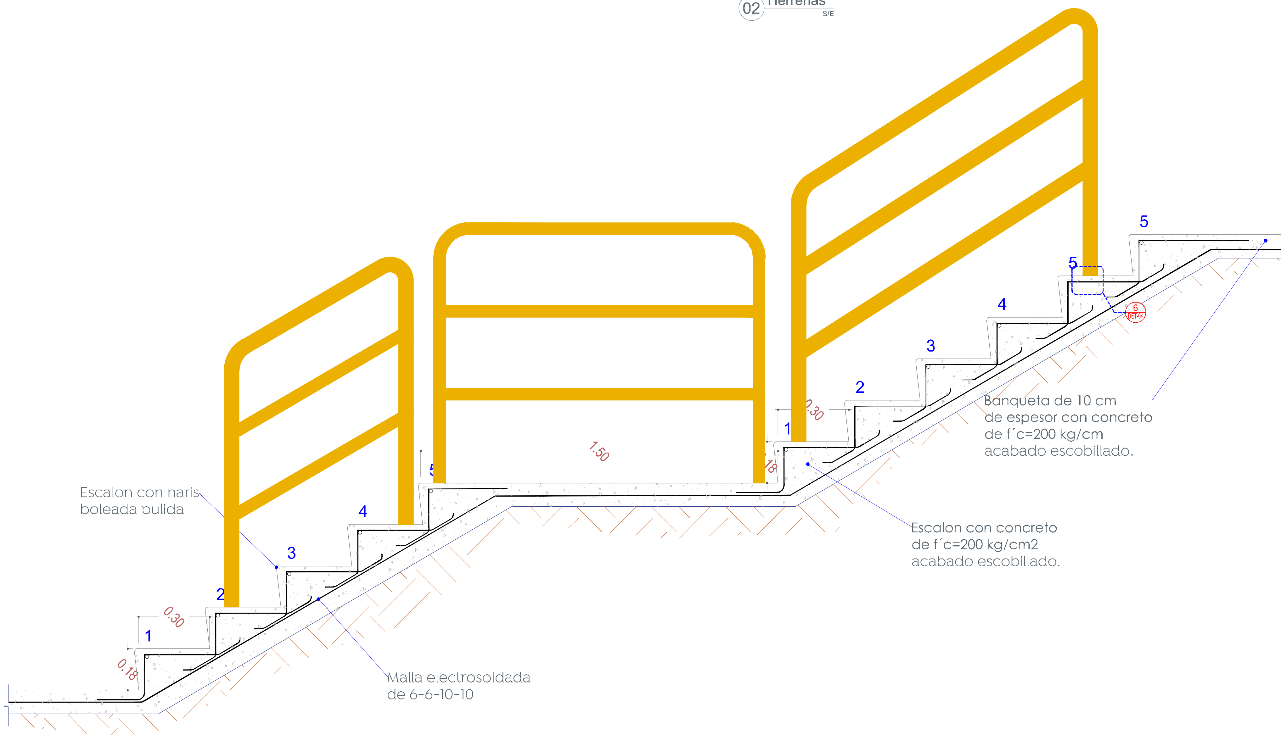
03 Seccion escalera S/E
