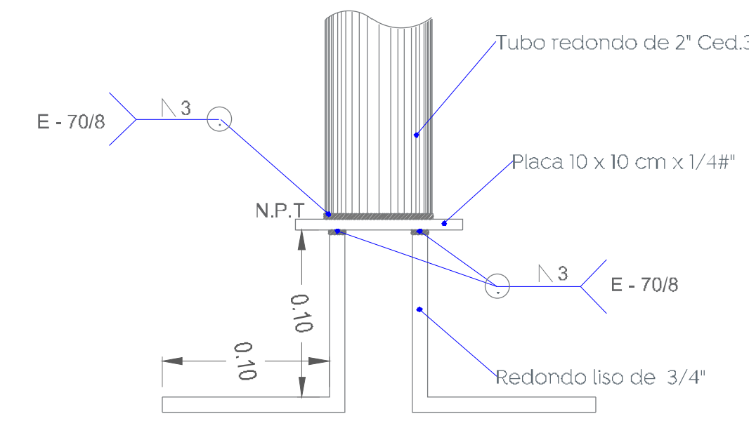
04 Soldadura de barandal S/E
