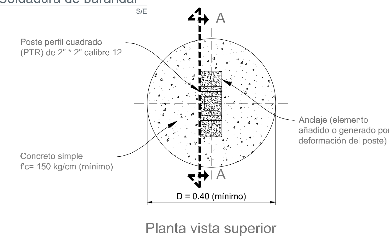
04 Soldadura de barandal S/E
