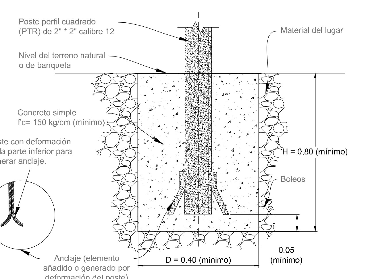
04 Dado de cimentación señalamiento vertical S/E
