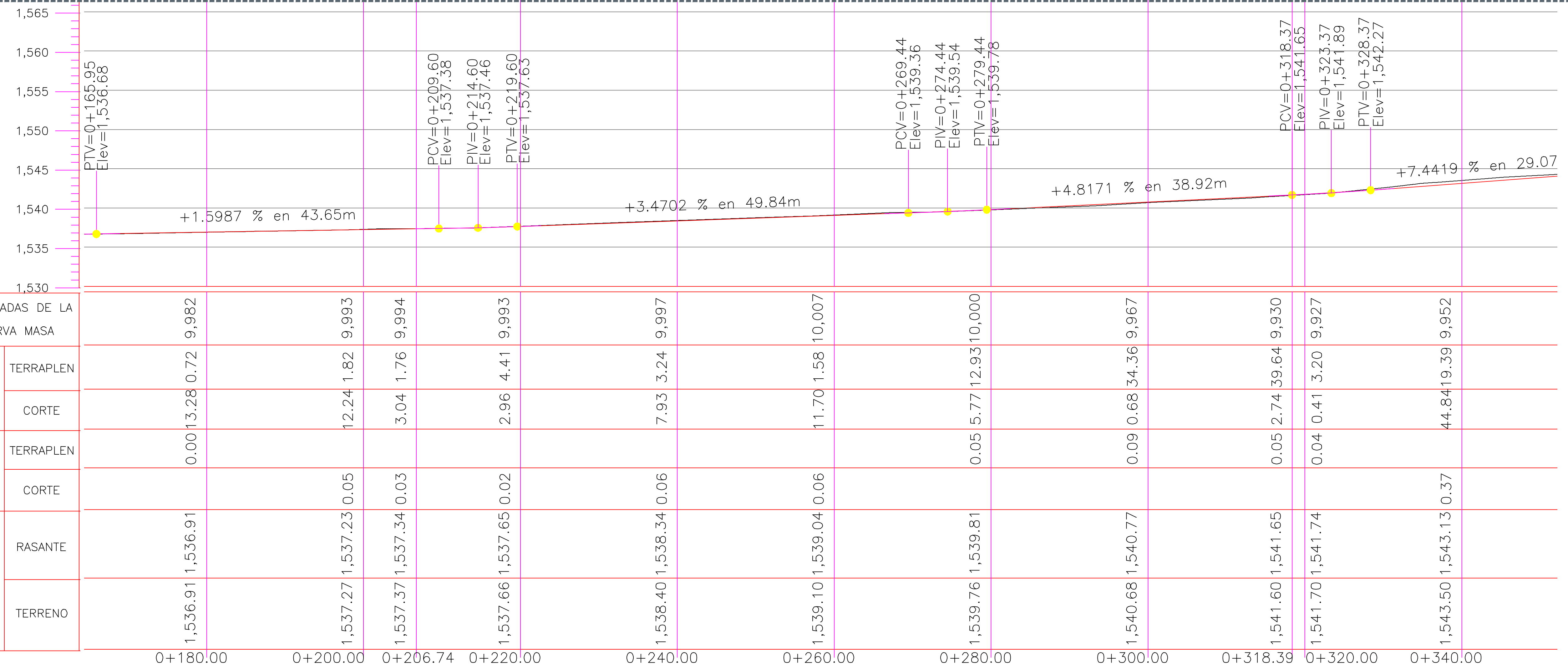
2 Perfil 0+180.00 a 0+340.00 Escala: 1:300
