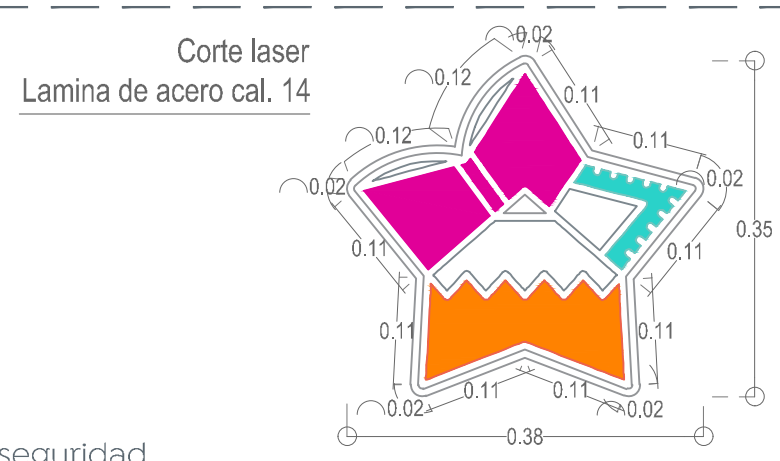
04 Barrera de seguridad
