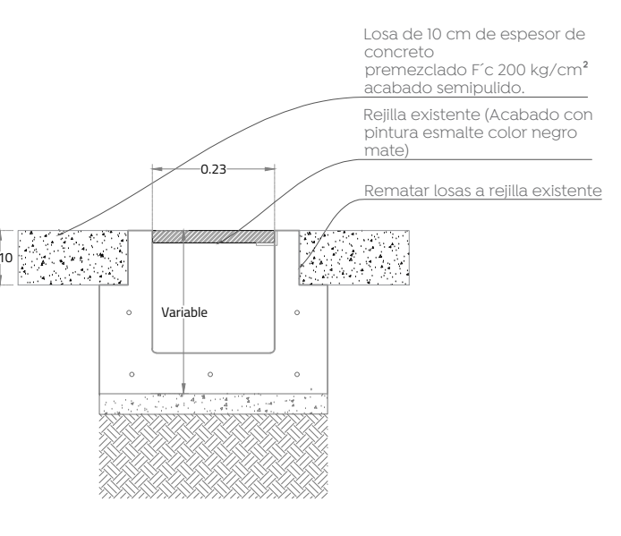
Detalle rejilla existente Detalles 1:20
