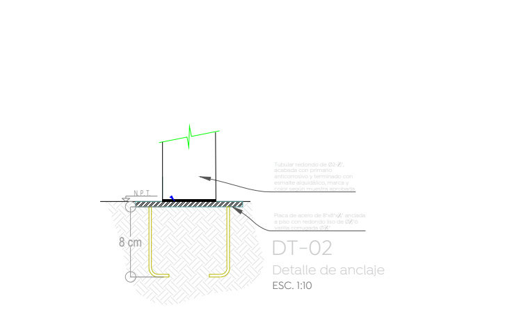
05 Detalle barandal Detalle anclaje barandal 1:10
