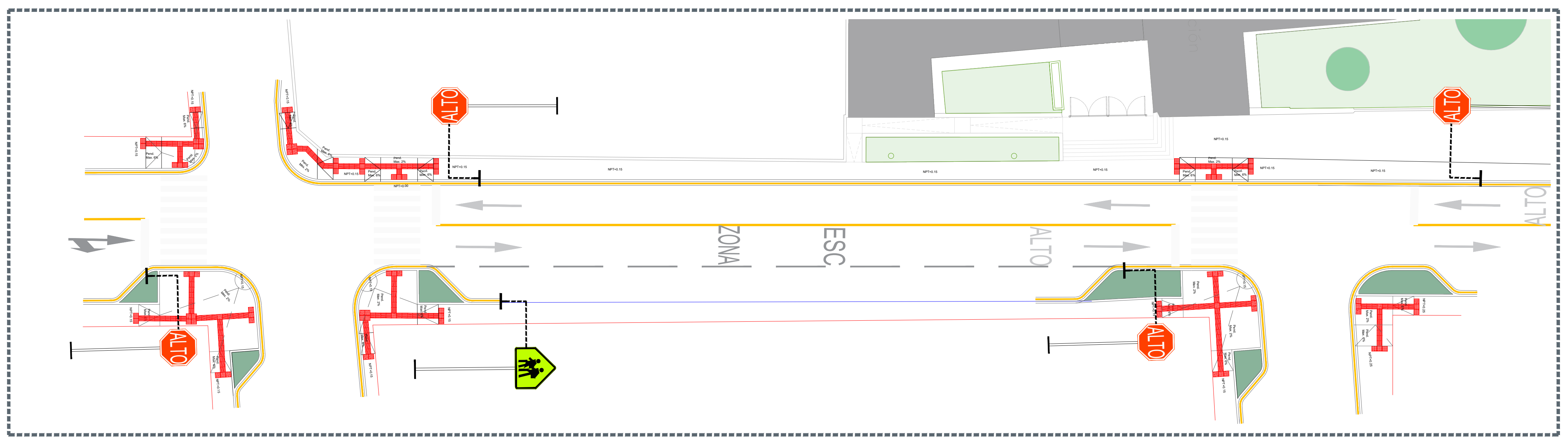
01 Planta general Escala 1:200
