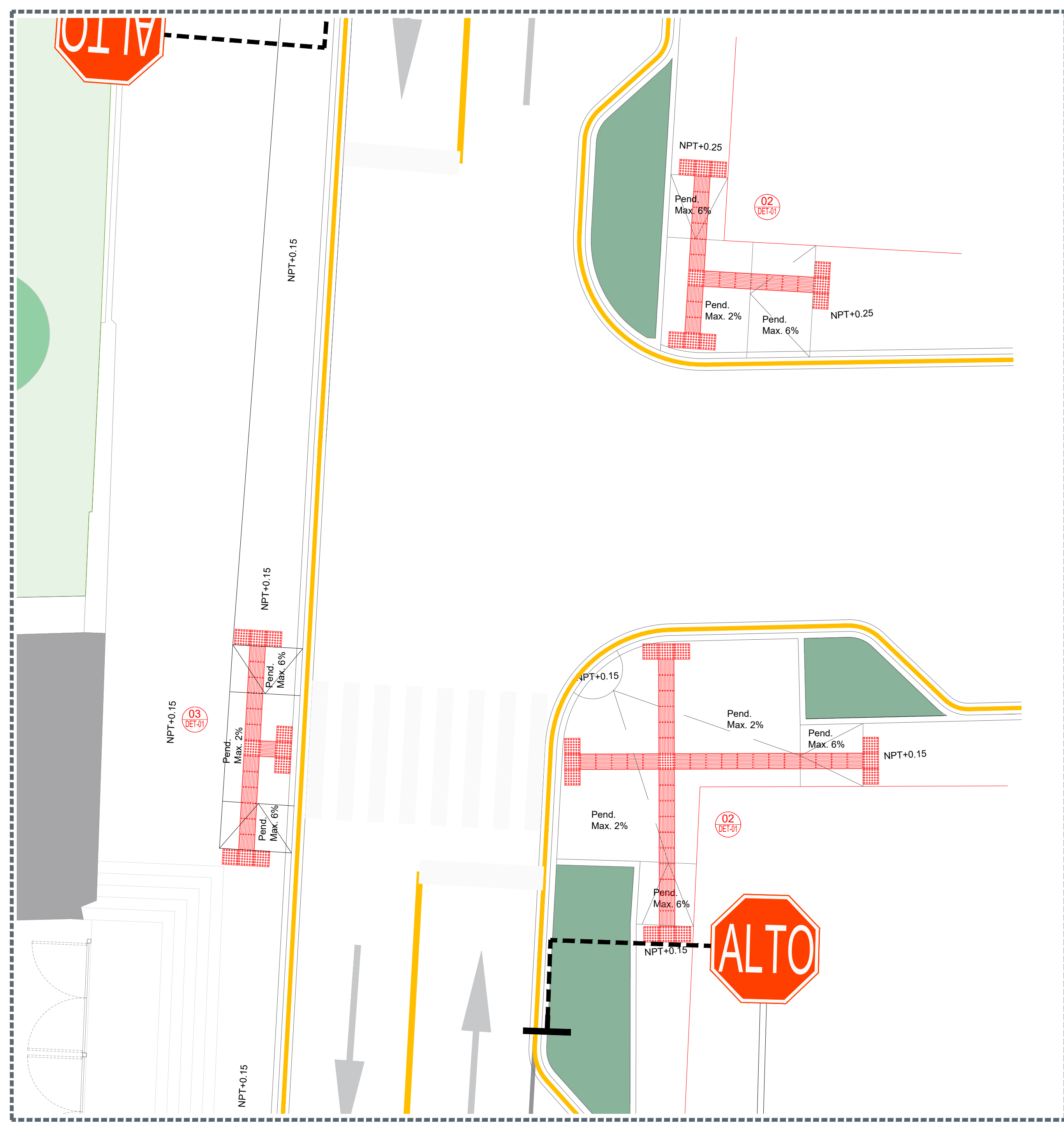
03 Crucero Seguro Escala 1:75
