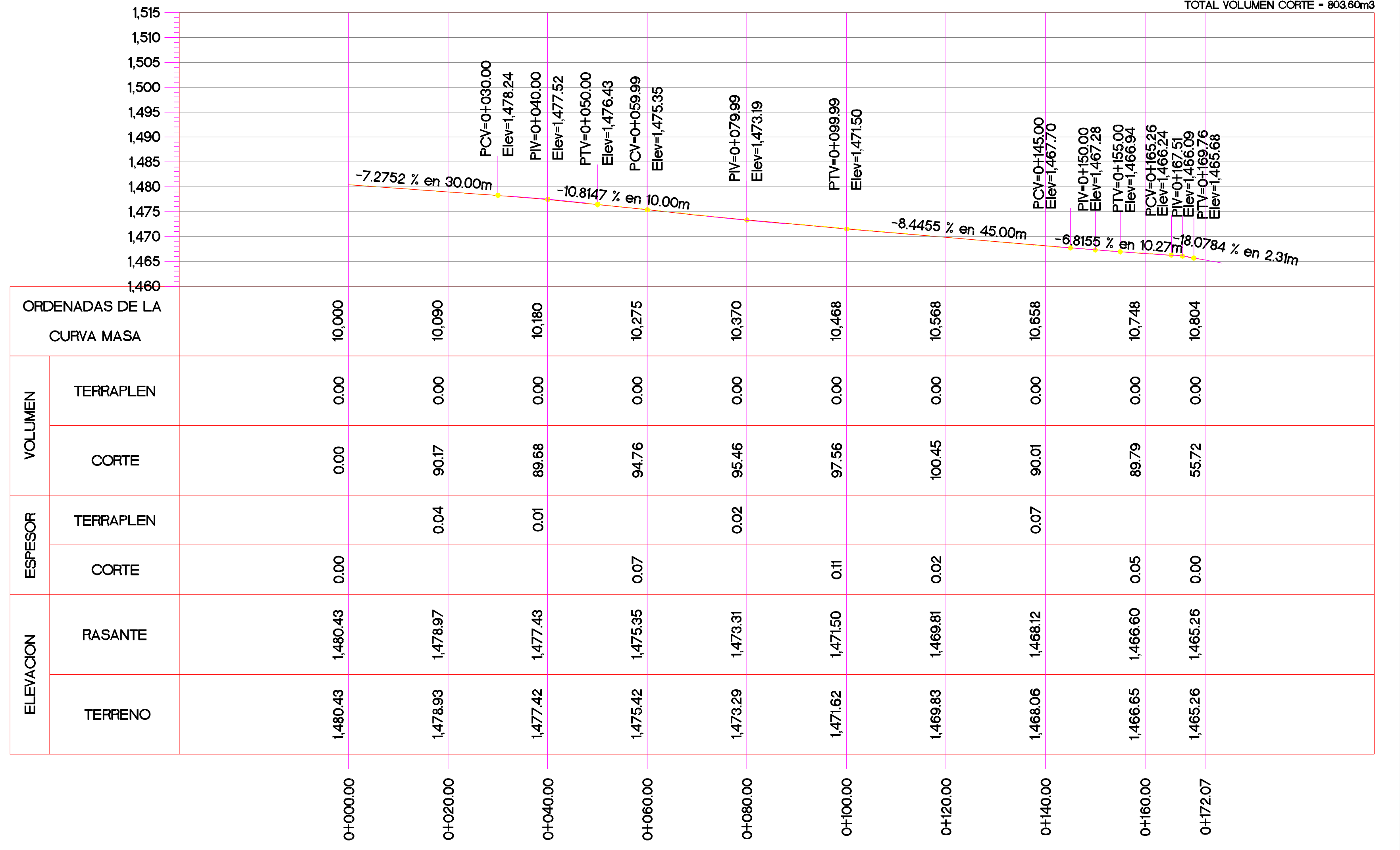
PERFIL Diamante ESCALA HORIZONTAL 1: 600 ESCALA VERTICAL 1: 600 TOTAL VOLUMEN CORTE = 803.60m 3
