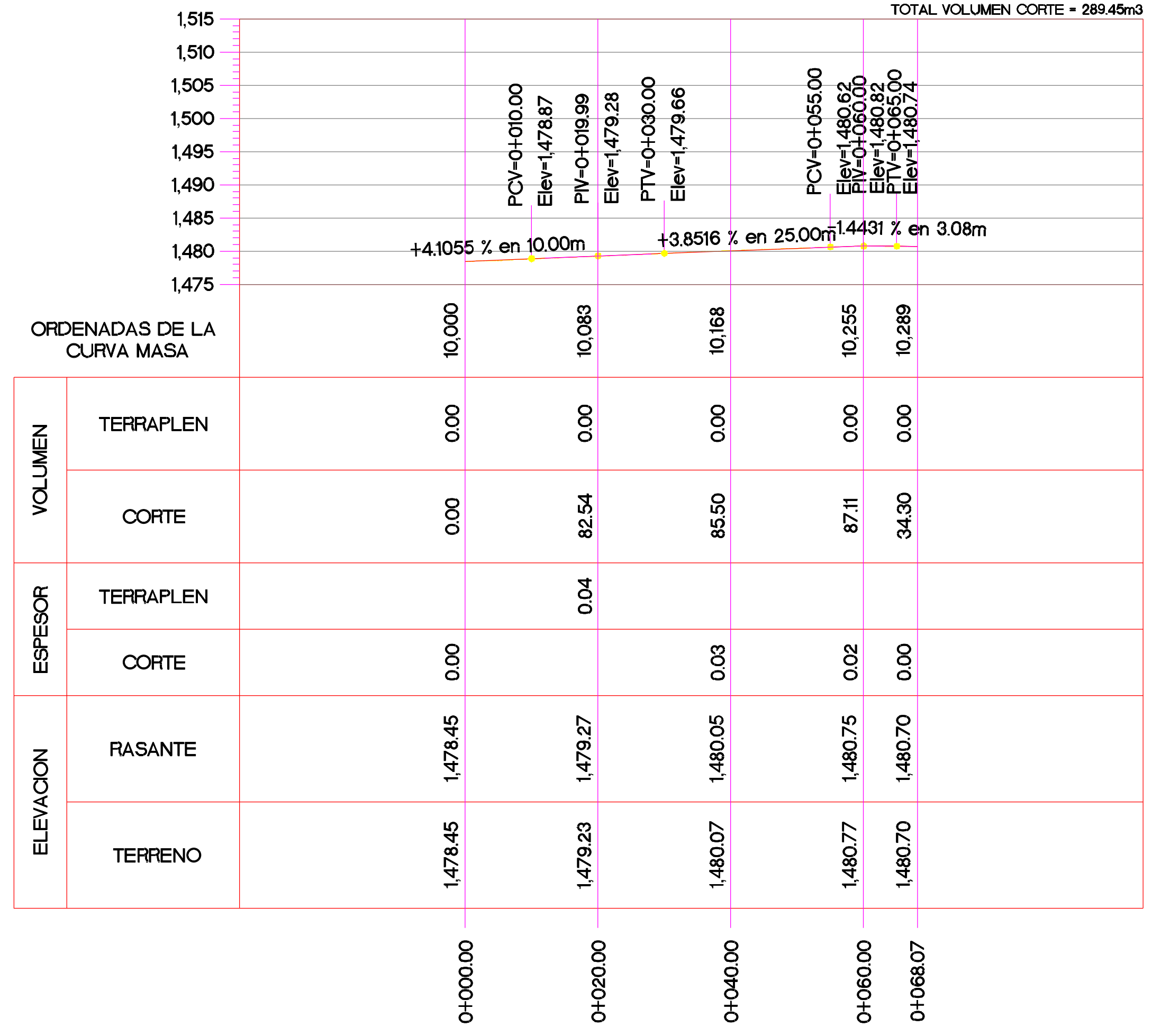
PERFIL Piedra Lisa ESCALA HORIZONTAL 1: 600 ESCALA VERTICAL 1: 600 TOTAL VOLUMEN CORTE = 289.45m 3
