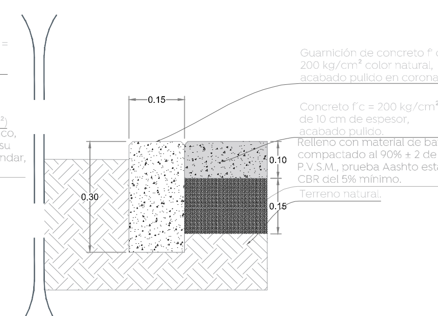
06 5. Concreto pulido Acabados 1:10
