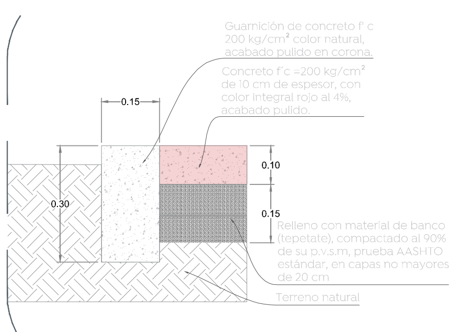
02 1. Concreto con color integral rojo Acabados 1:10
