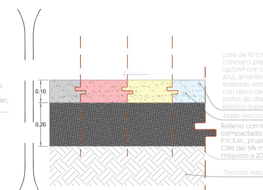
07 6. Concreto en cancha de usos múltiples Acabados 1:10
