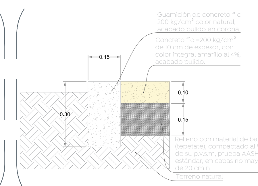
04 3. Concreto con color integral amarillo Acabados 1:10
