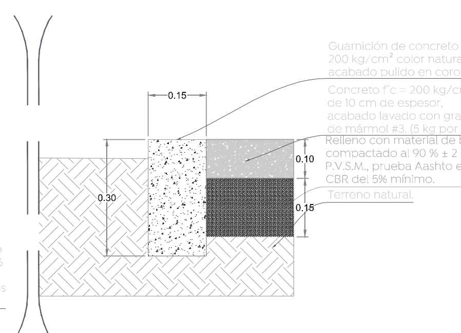
05 4. Concreto lavado Acabados 1:10
