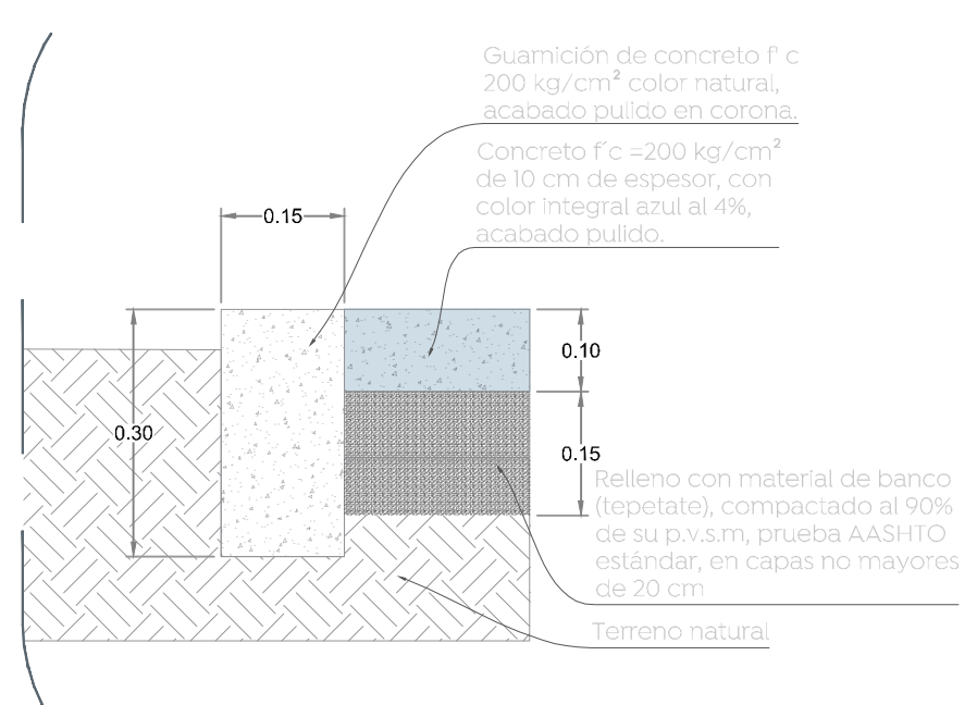
03 2. Concreto con color integral azul Acabados 1:10
