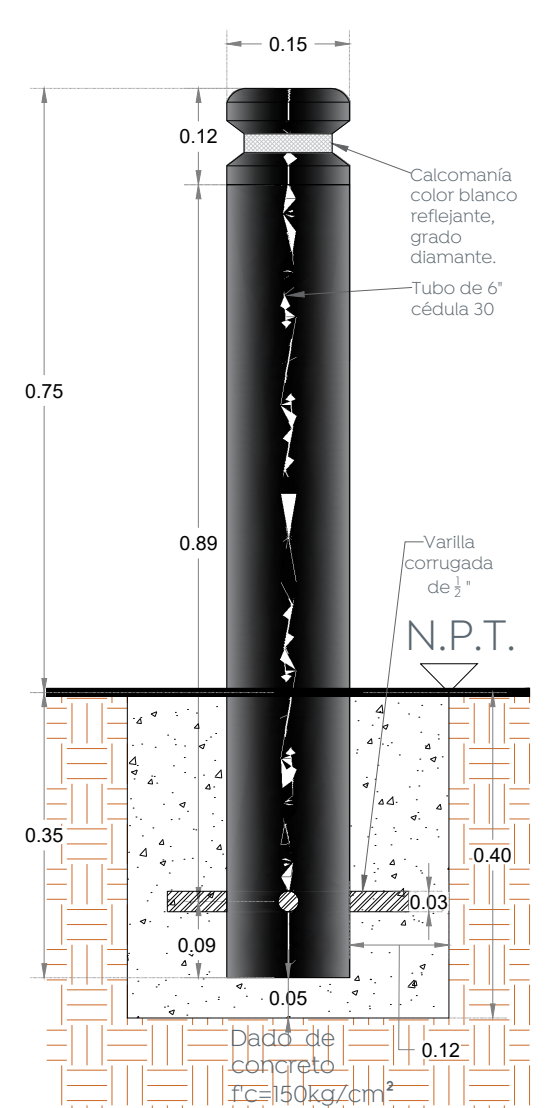
Detalle de bolardo 2 Pm
