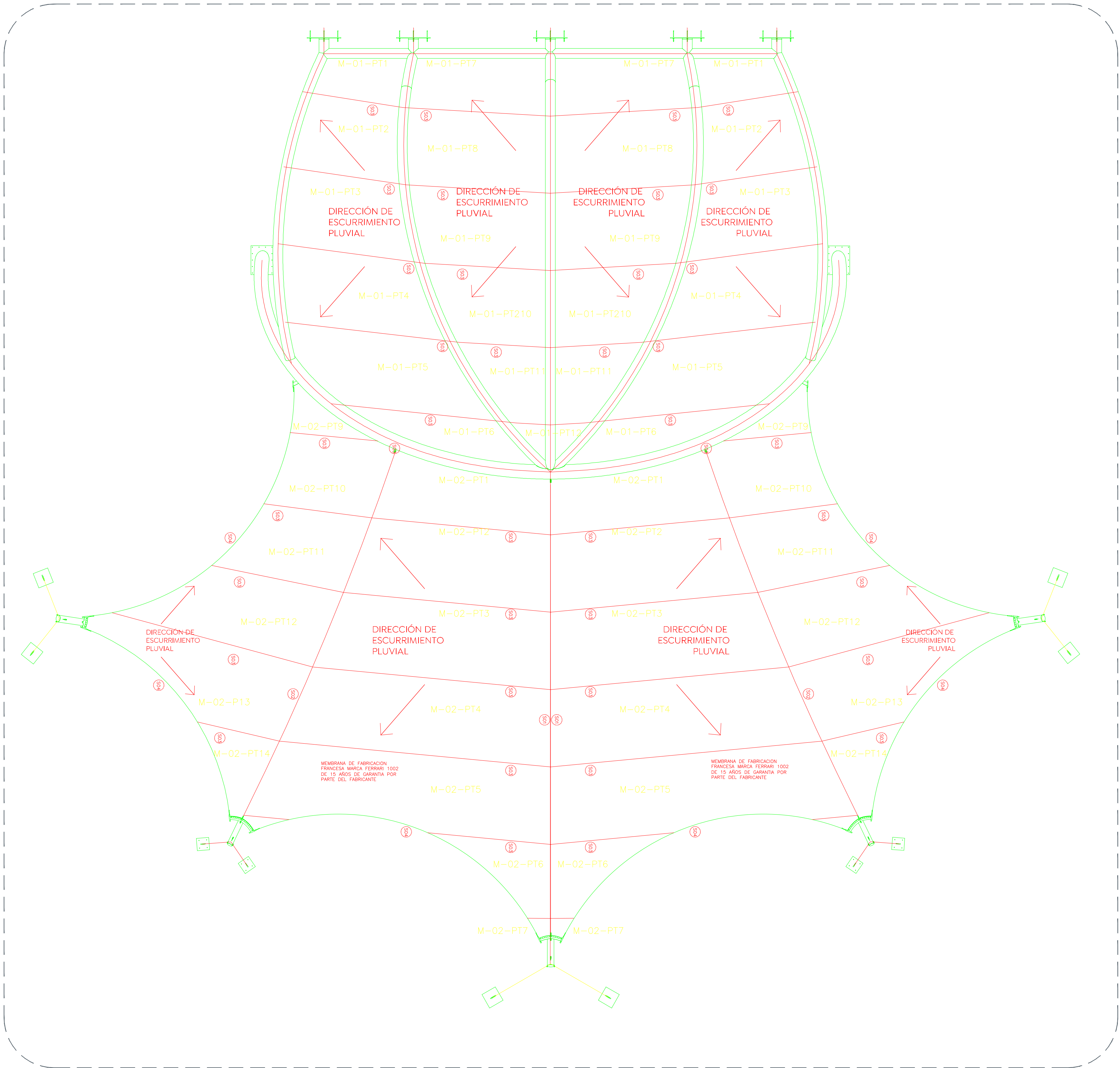
01 Patronaje de membrana Agora - Parque De Las Niñas y Los Niños 1:75
