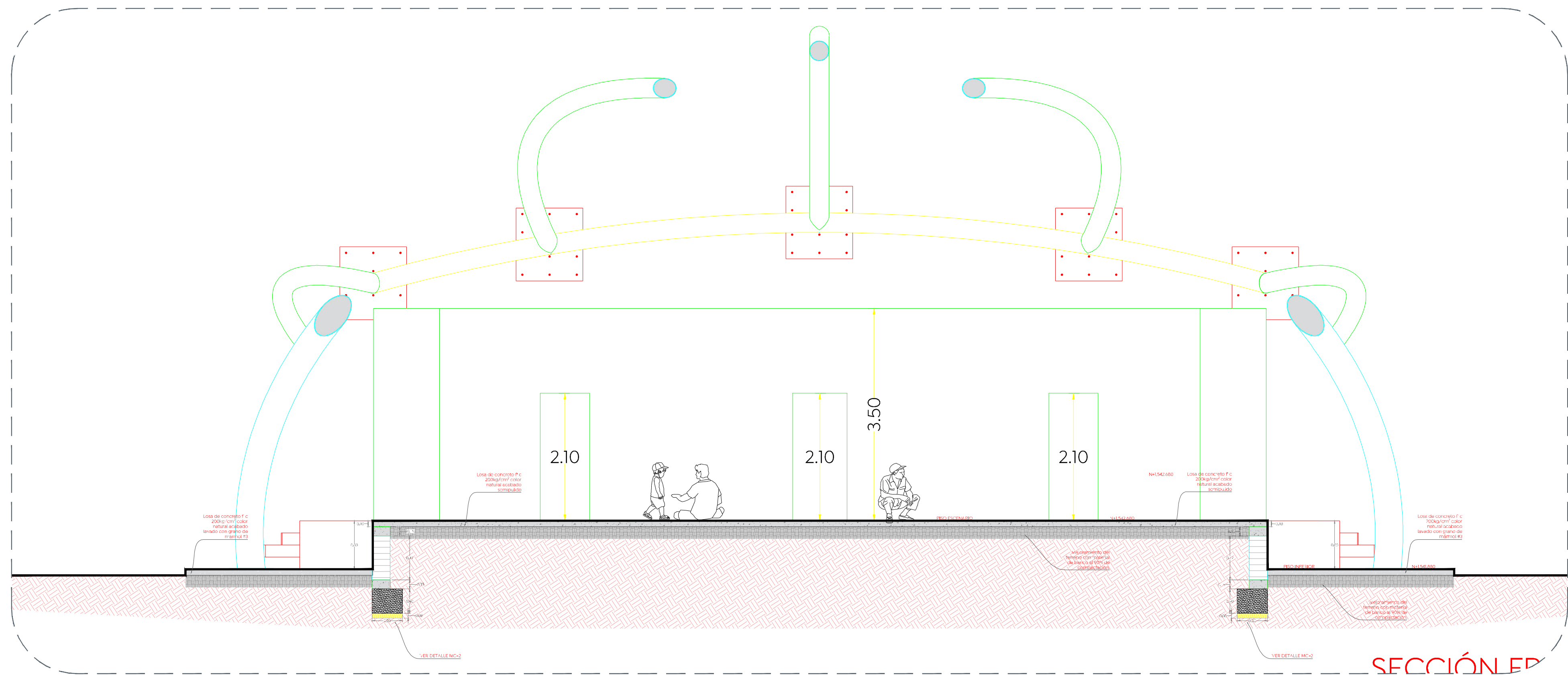
01 Sección frontal escenario Ágora - Parque De Las Niñas y Los Niños 1:50
