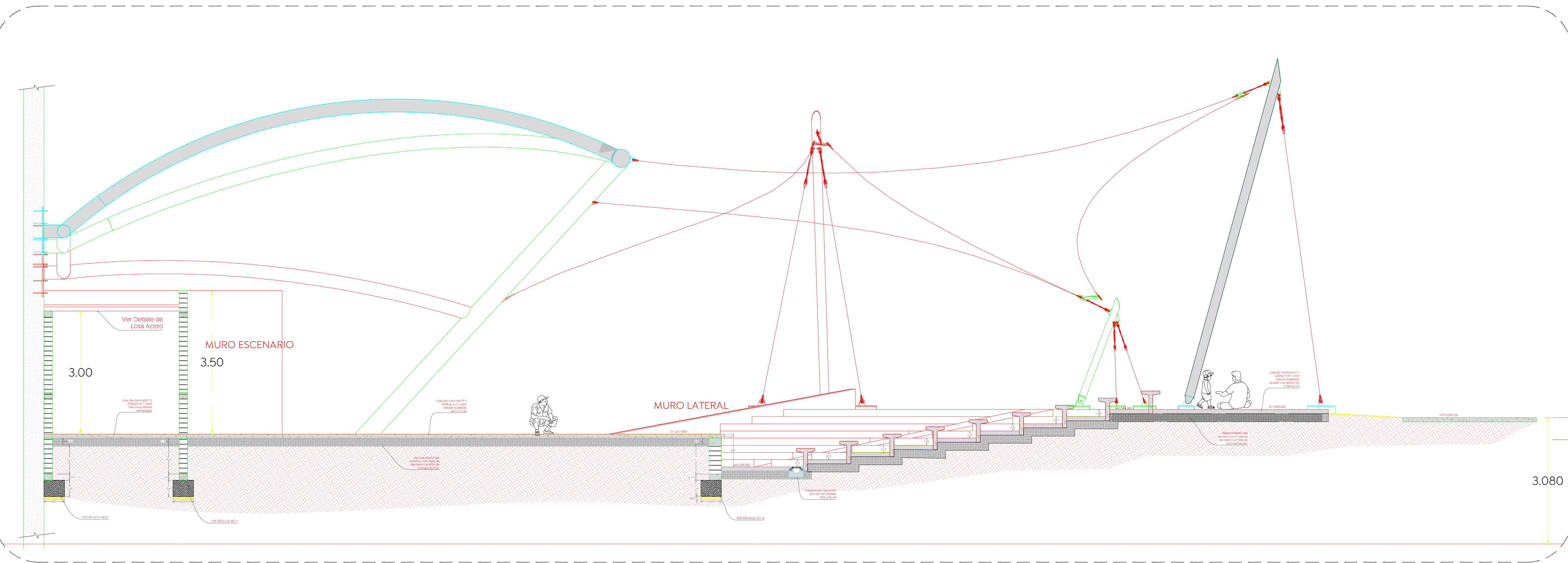
02 Sección longitudinal Ágora - Parque De Las Niñas y Los Niños 1:50
