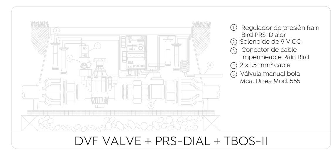
03 Detalle Válvula Solenoide S/E
