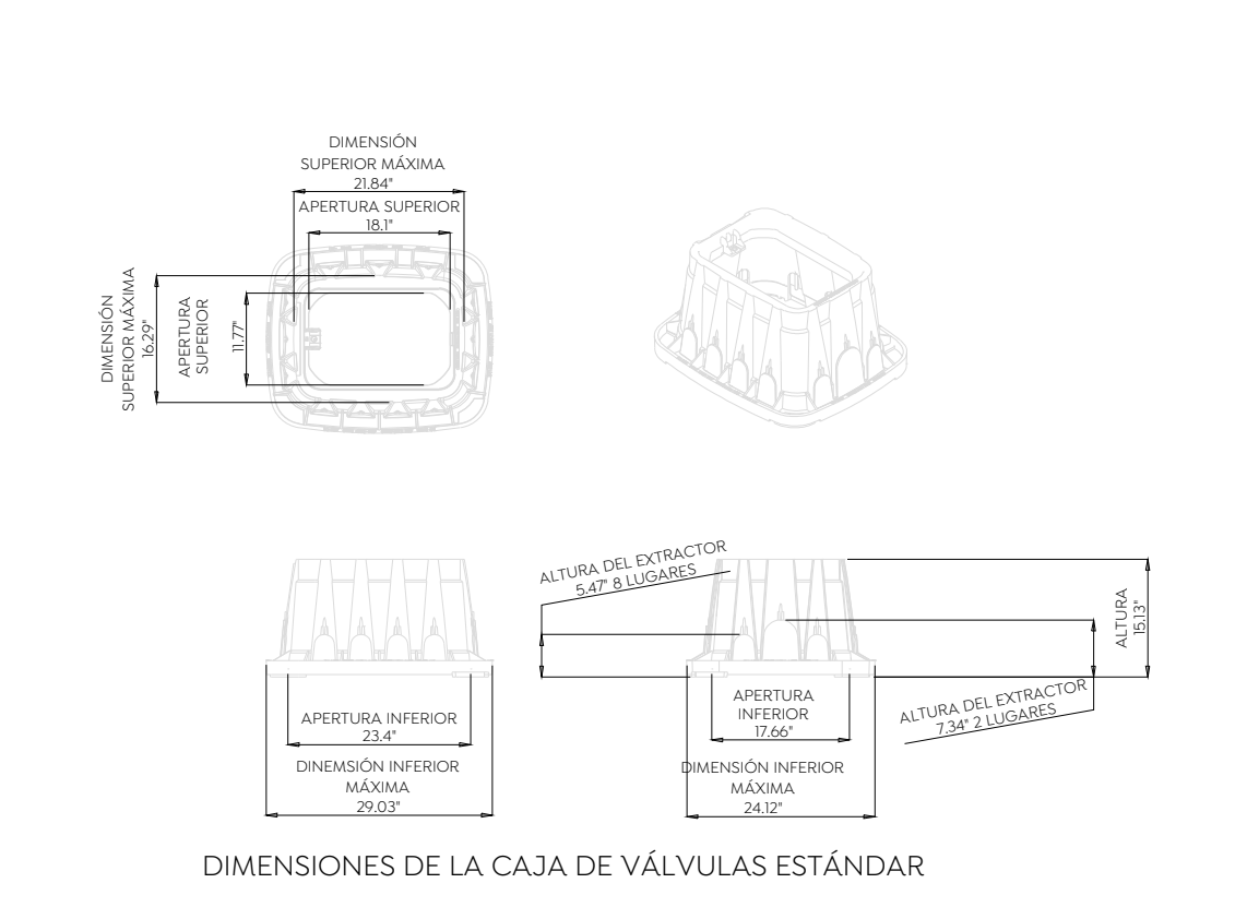
04 Detalle Caja de Válvulas S/E
