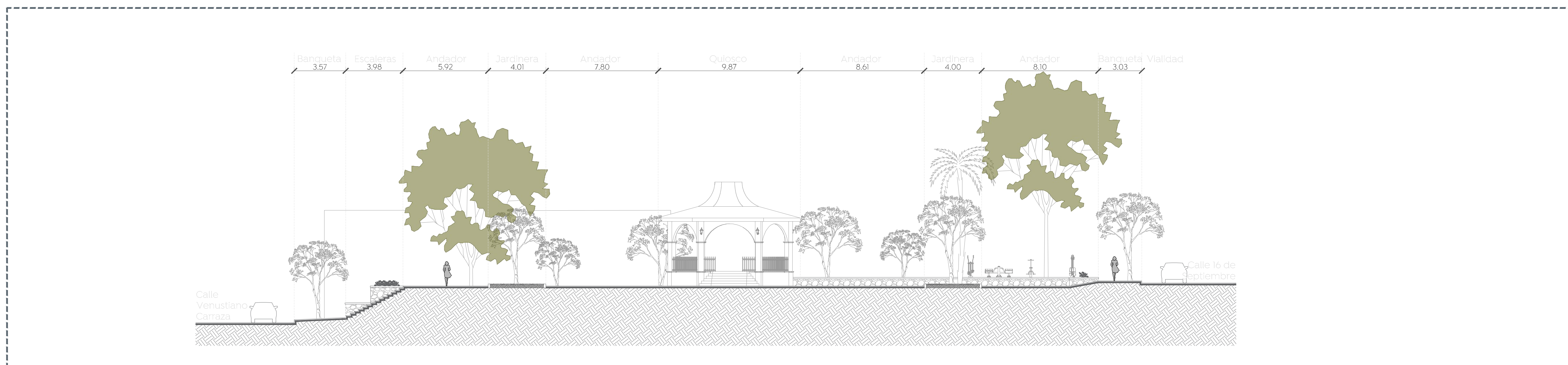
02 Sección B - B'
