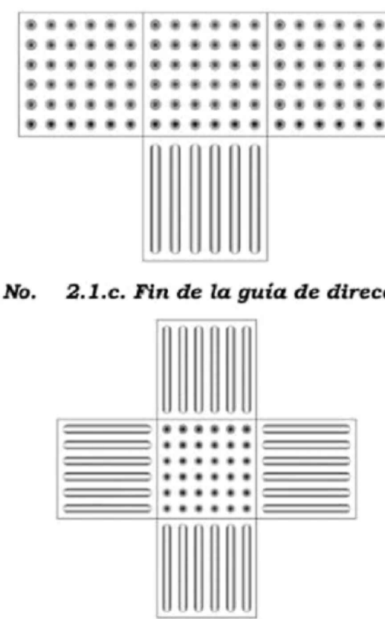
Figura No. 2.1.d. Cambios de dirección.
