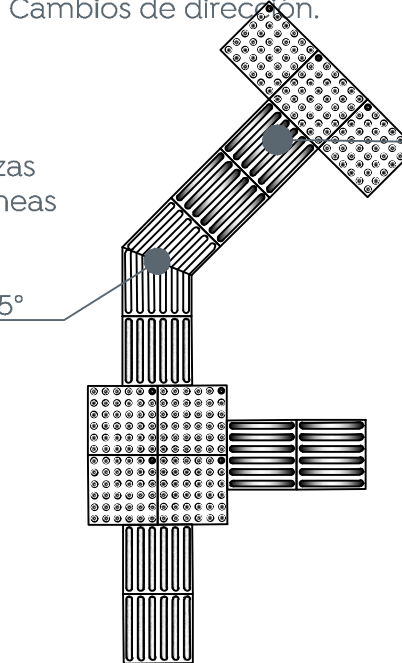
Figura No. 2.1.d. Cambios de dirección.
