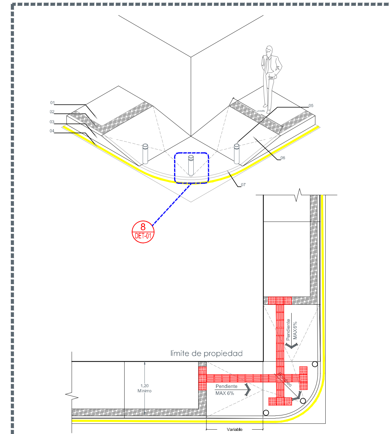
2.1 Detalle esquina S/E
