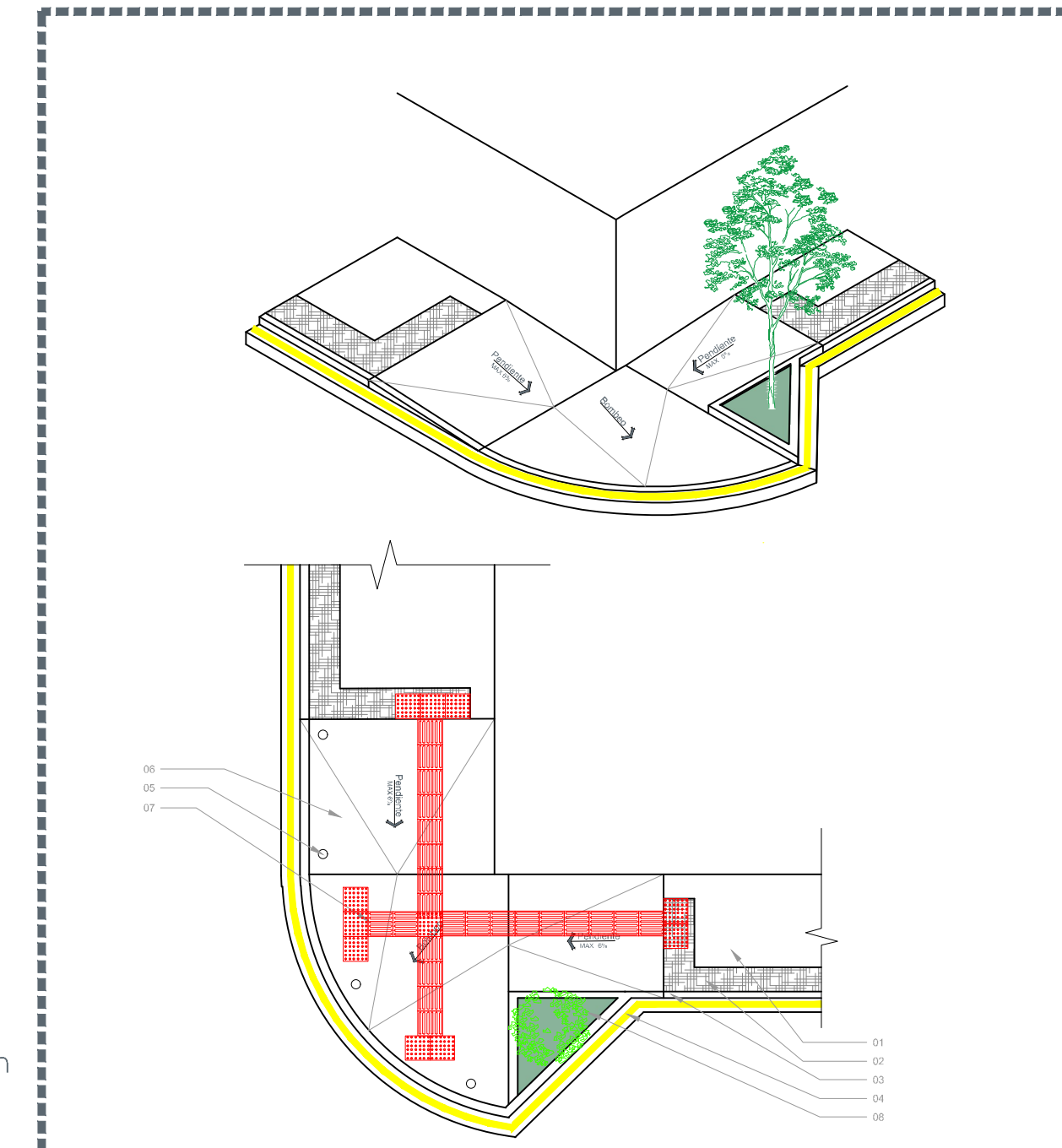
2.2 Esquina tipo con bahía S/E
