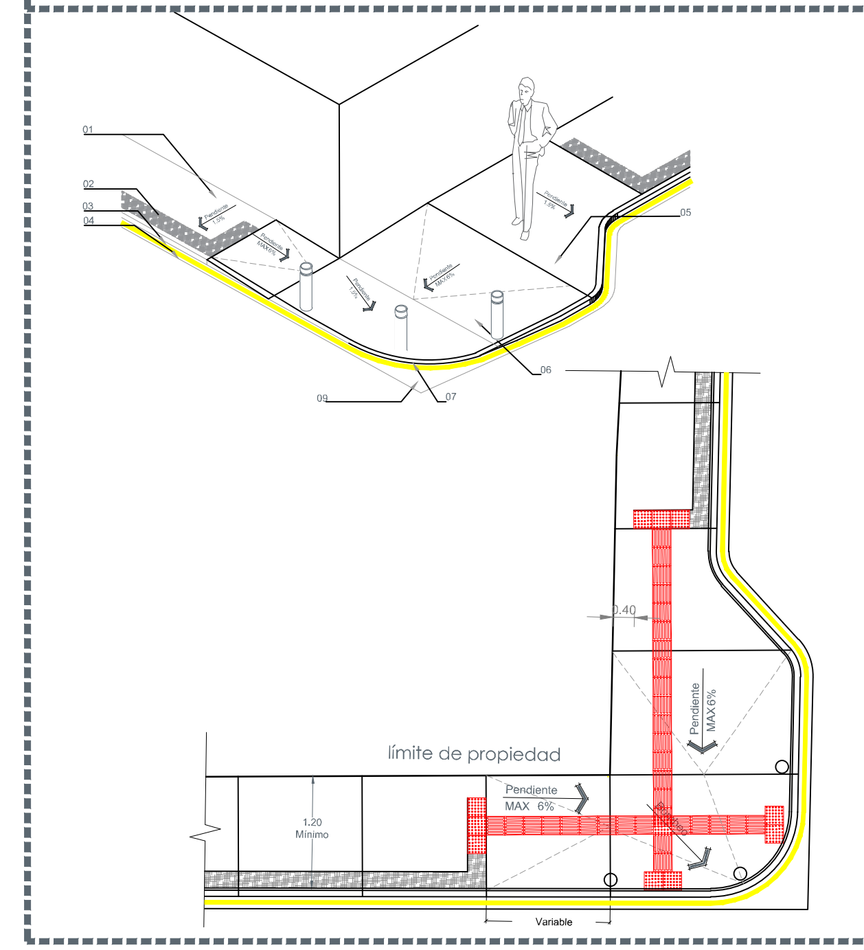
2.3 Esquina tipo con bahía S/E
