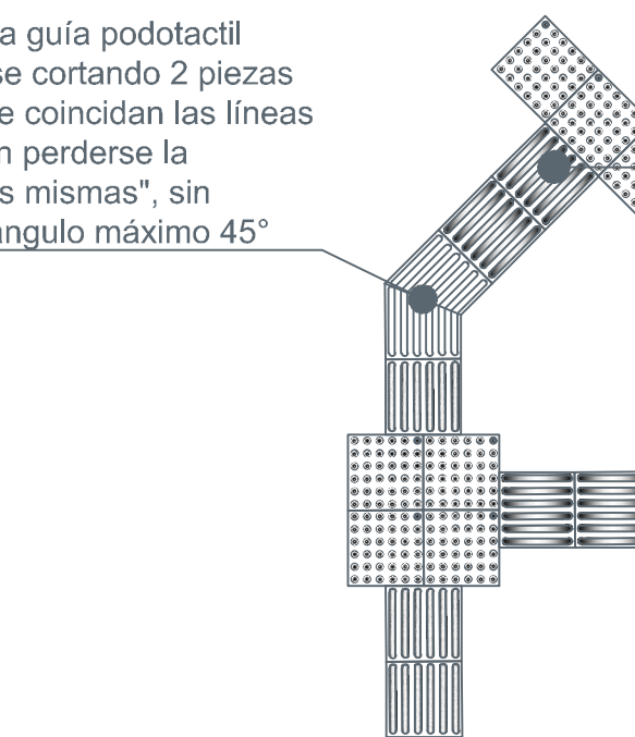
Figura No. 2.1.e. Cambios de dirección.
