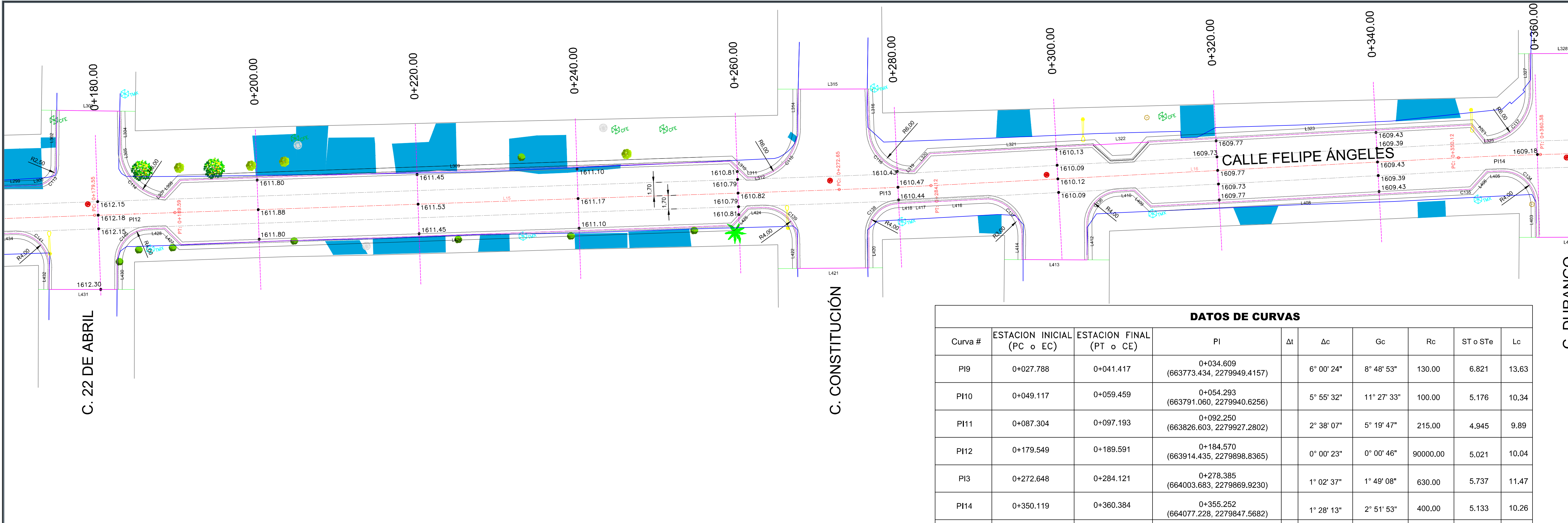
1 Planta general Escala 1:250
