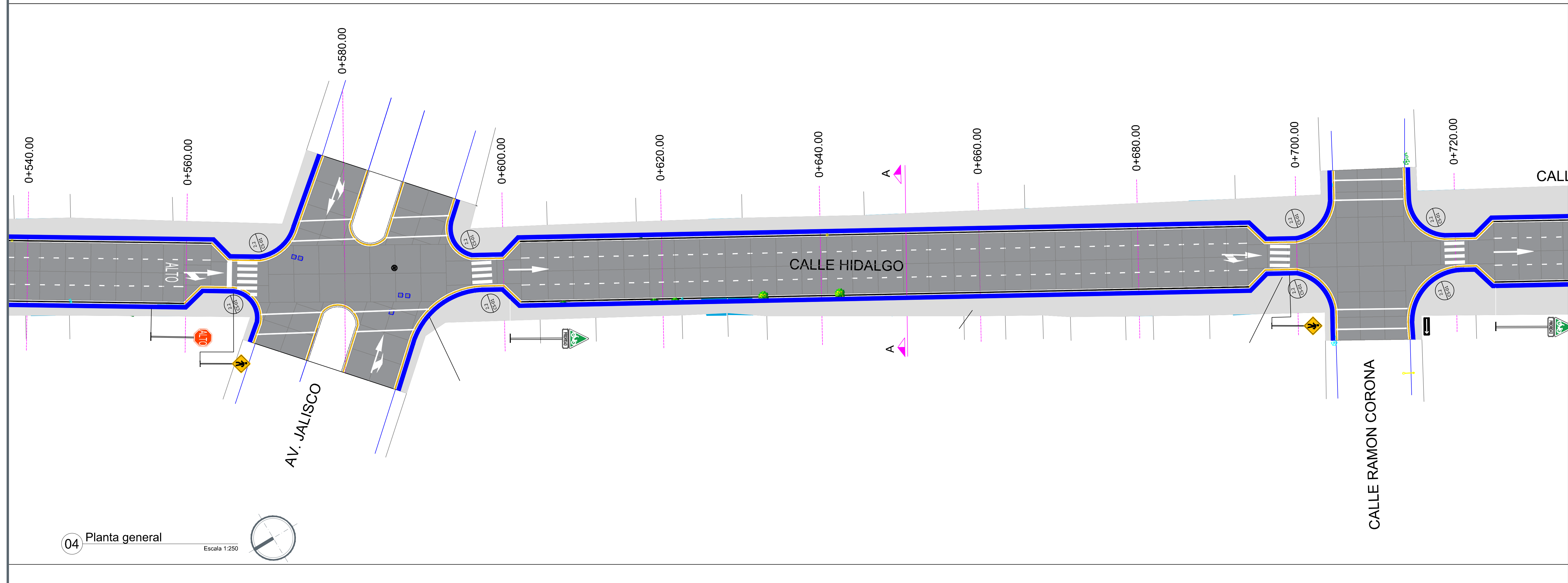
03 Planta general Escala 1:250
