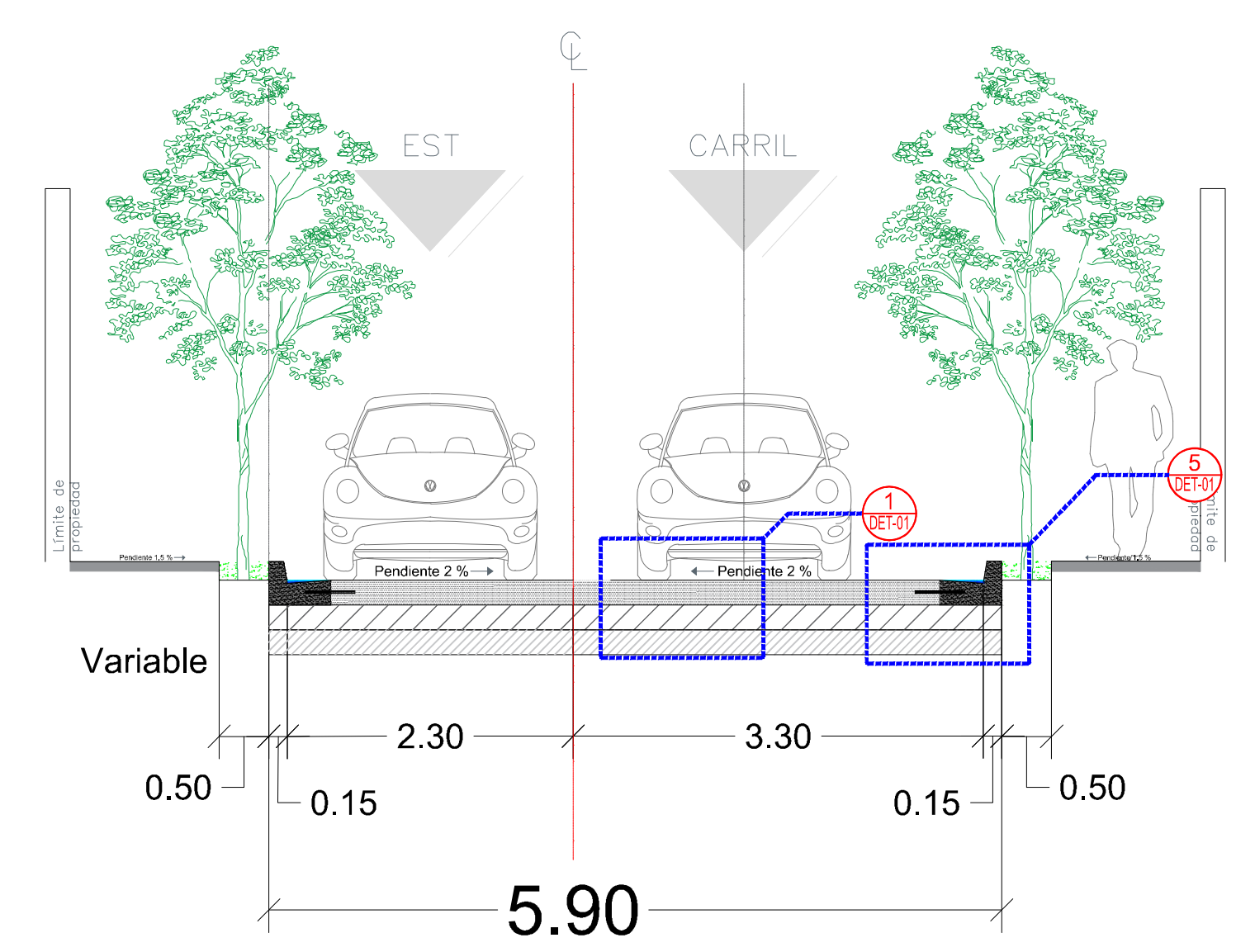
1 Seccion Escala 1:75
