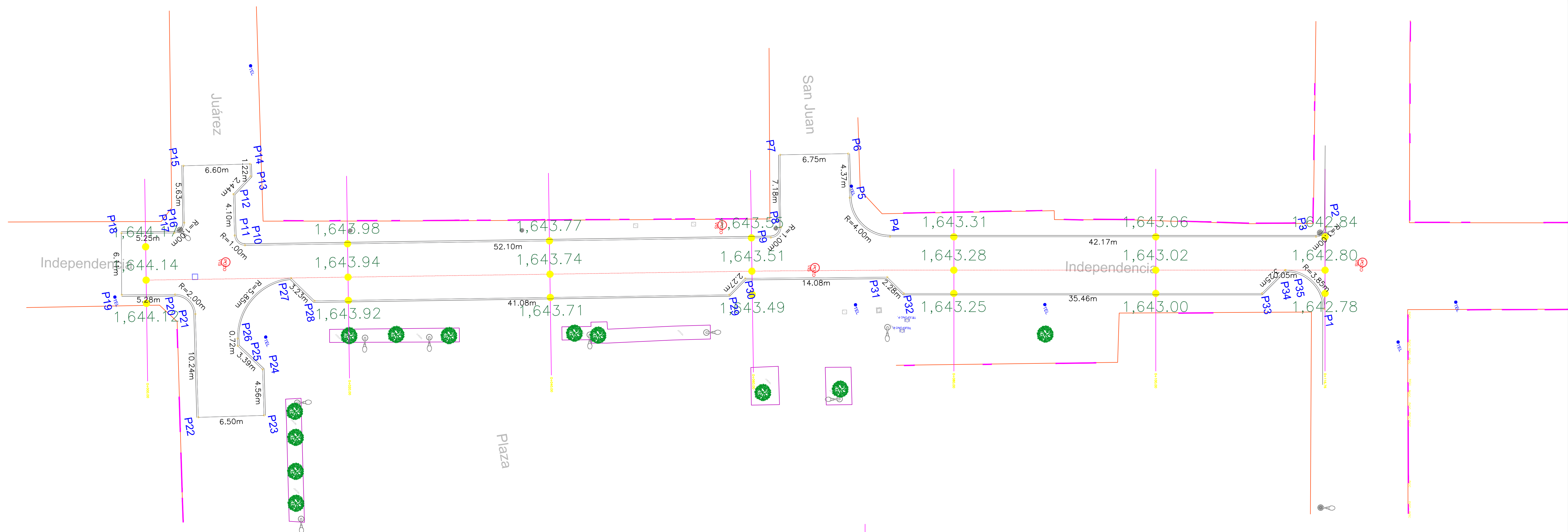
1 Planta de rasantes Escala 1:200
