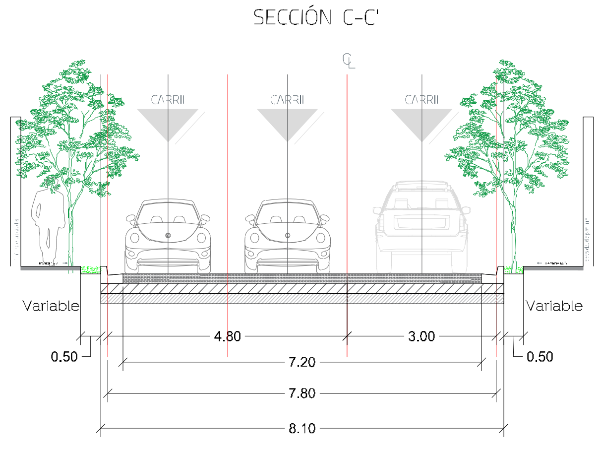
5 Secciones Escala 1:75
