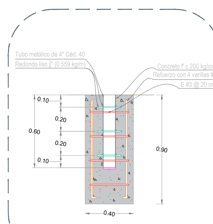
03 Anclaje portería de usos múltiples d1
