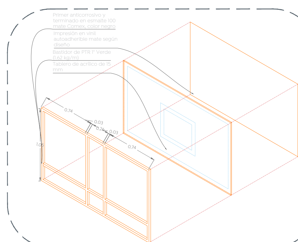
04 Detalle de tablero d1
