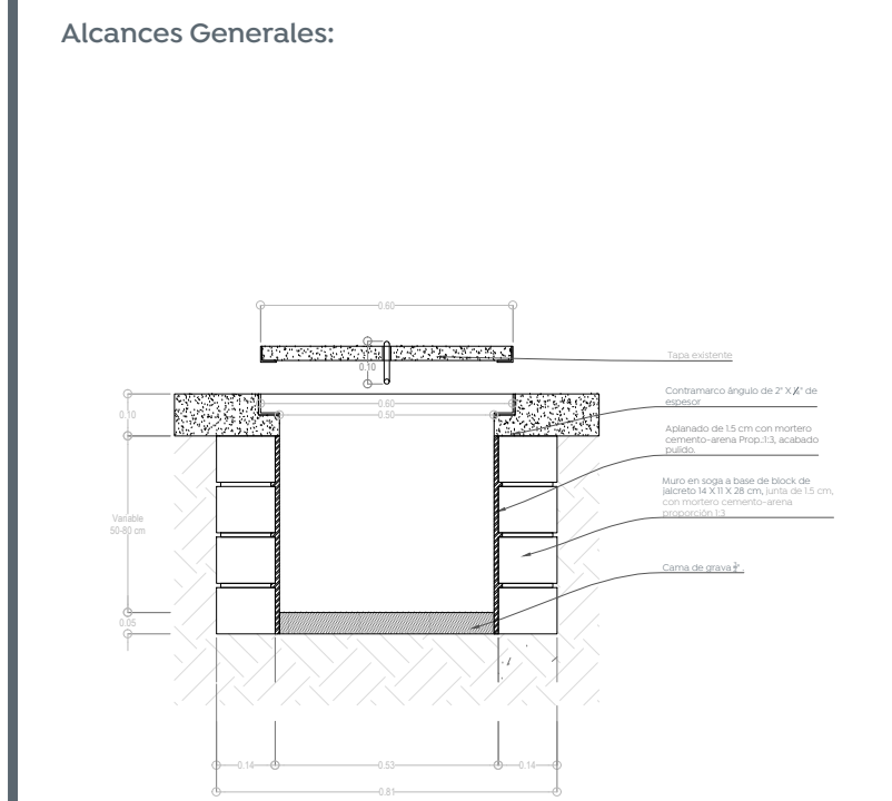
03 Detalle registro Acabados en piso 1:20
