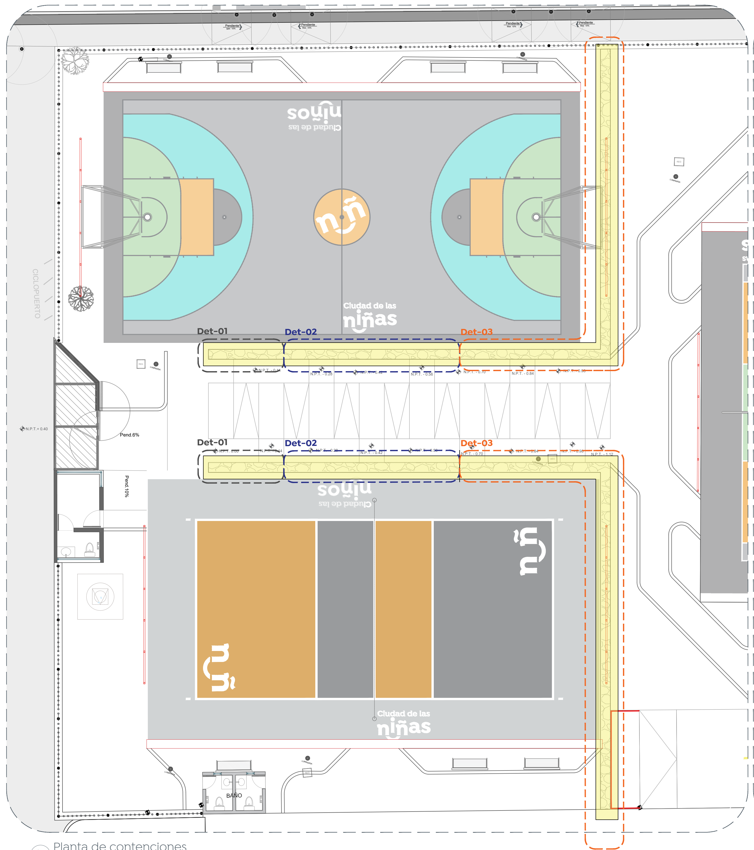
01 Planta de contenciones Mampostería 1:100
