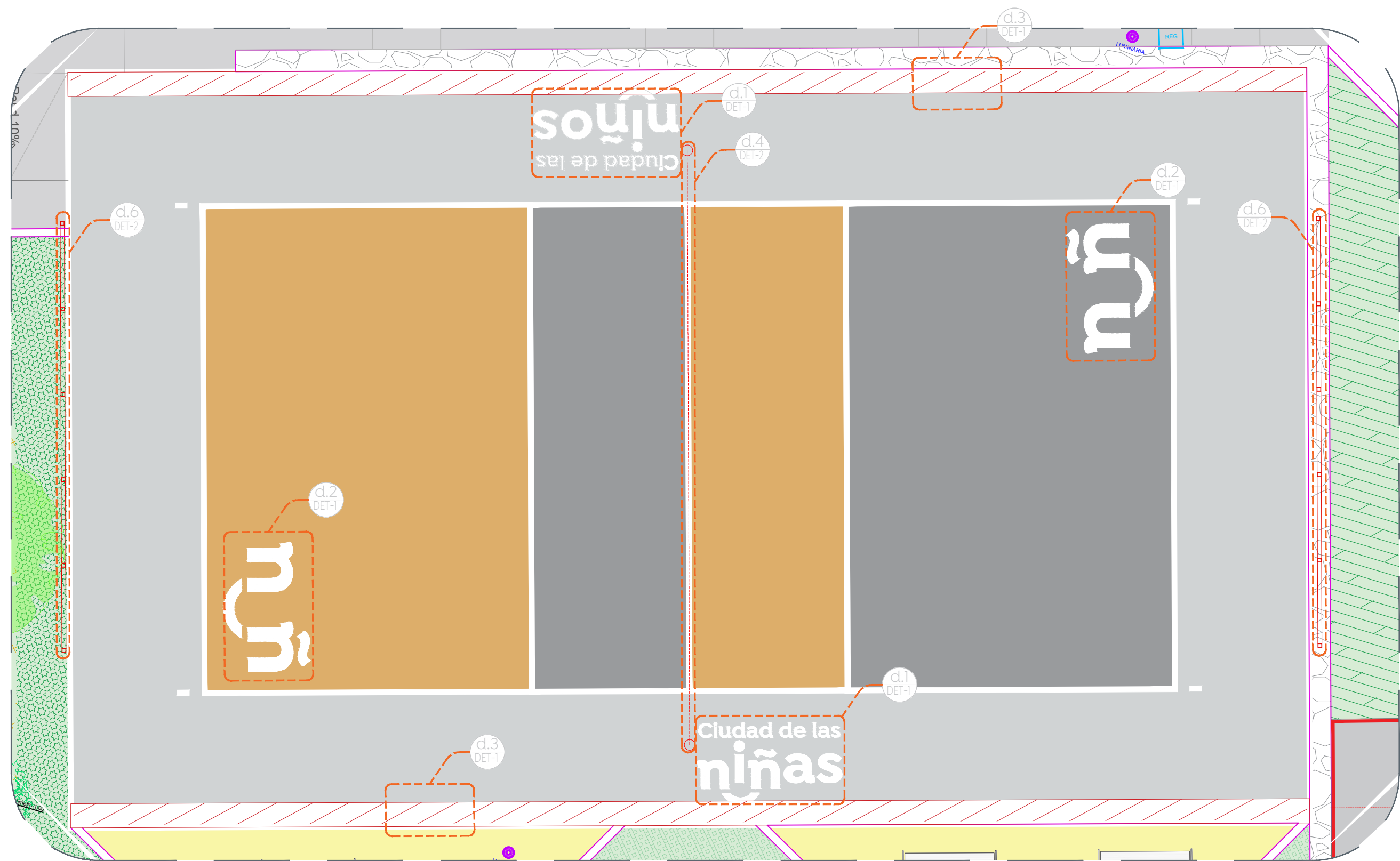
01 Planta cancha de voleibol Llamadas a detalles 1:75
