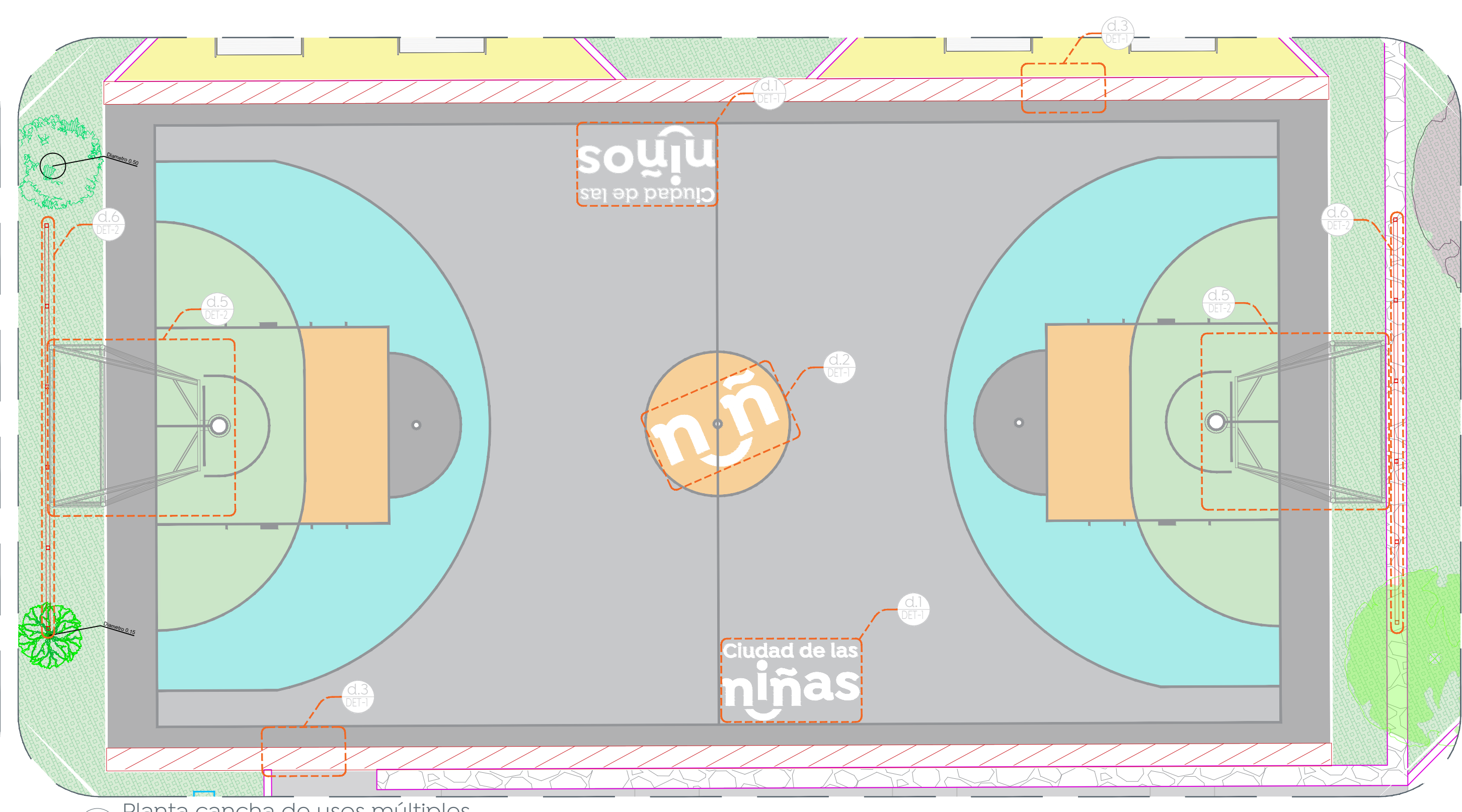
03 Planta cancha de usos múltiples Llamadas a detalles 1:75
