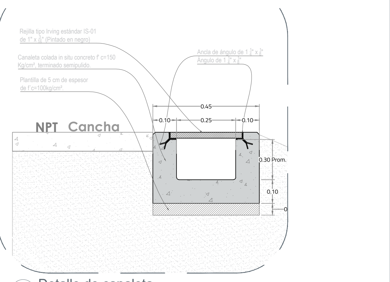
07 Detalle de canaleta d.3 1:10
