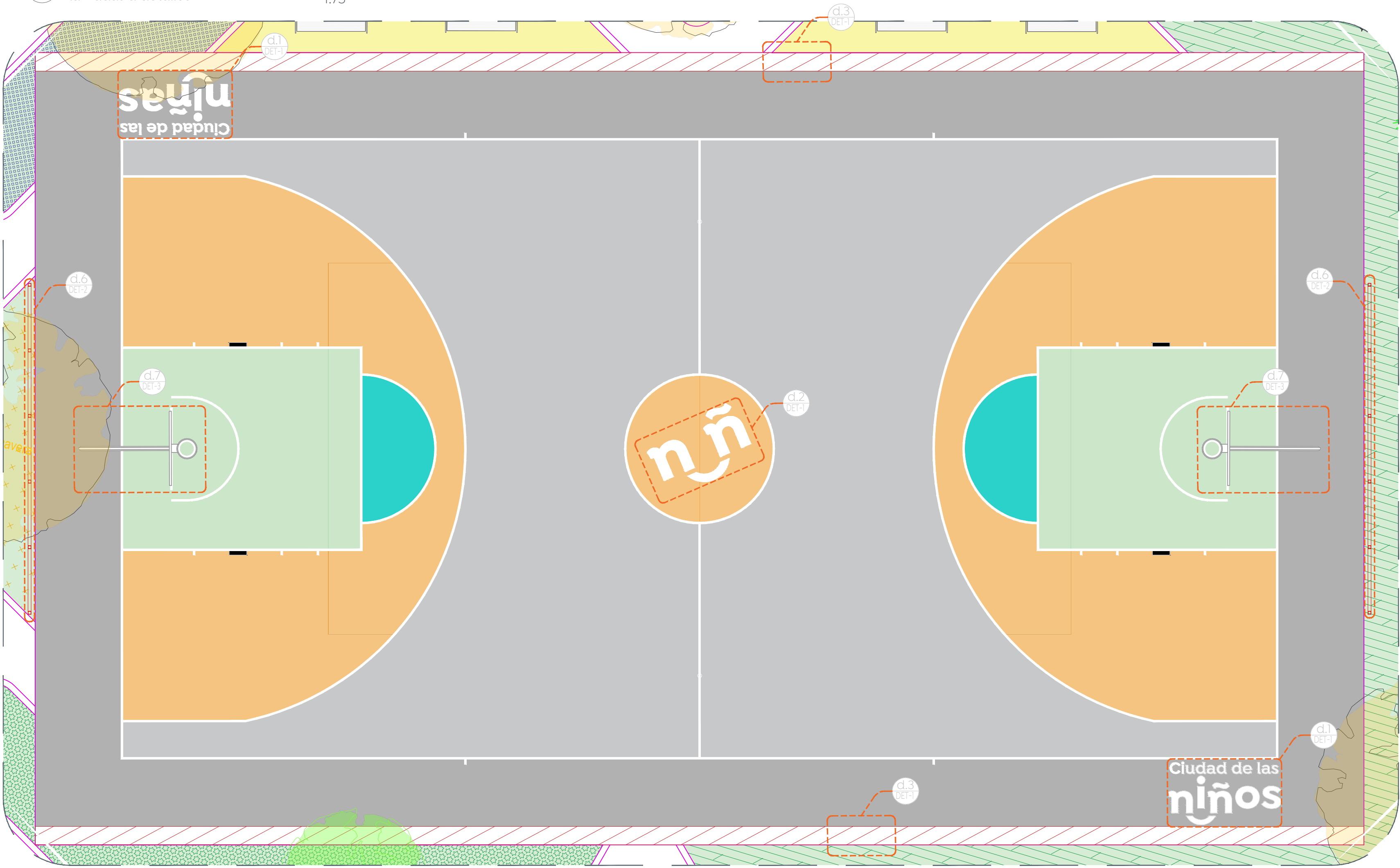
02 Planta cancha de básquetbol Llamadas a detalles 1:75
