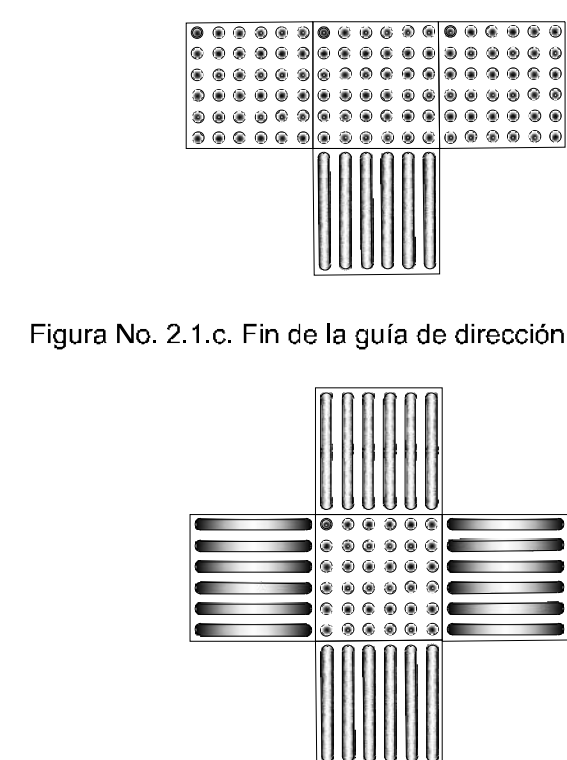
Figura No. 2.1.d. Cambios de dirección.
