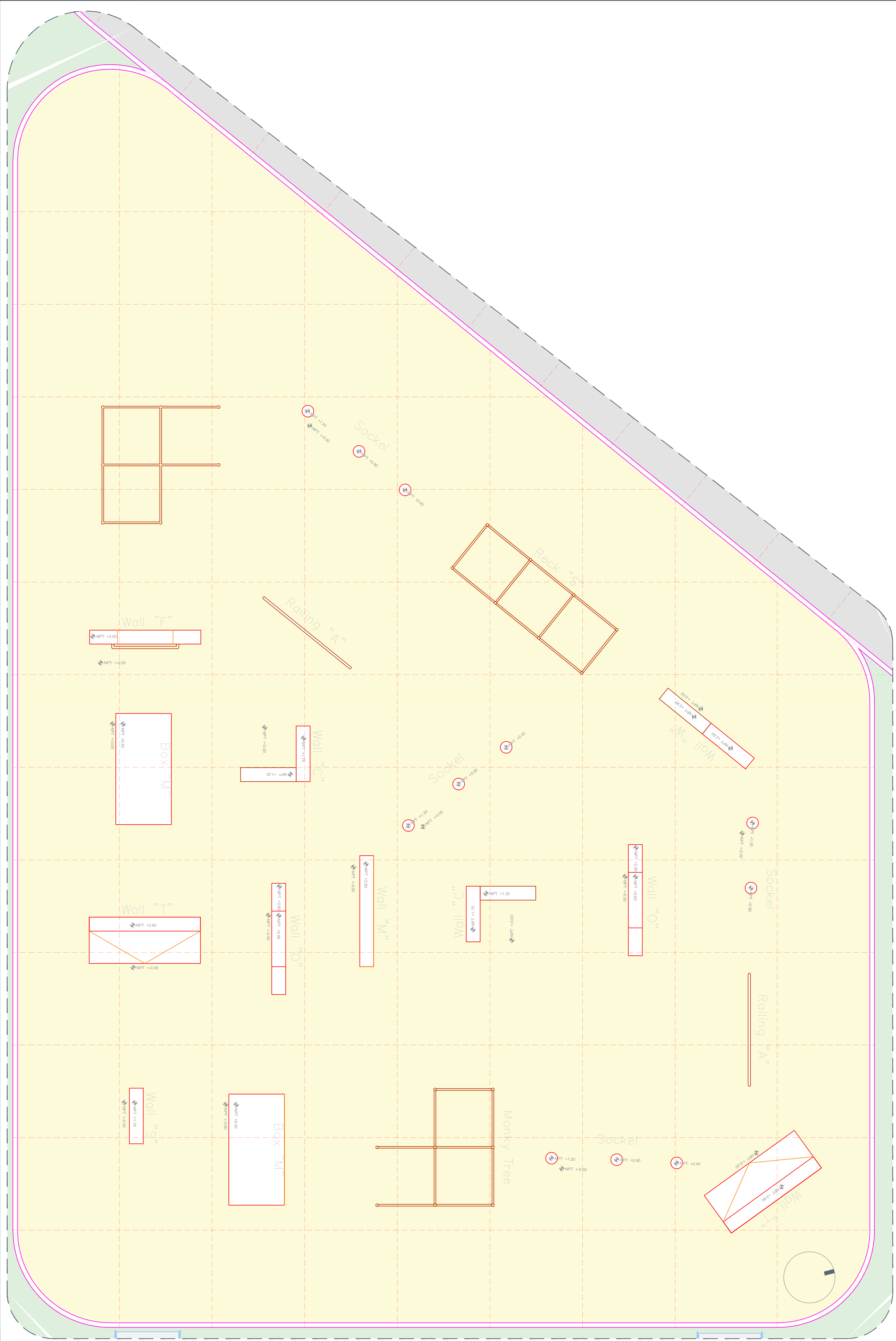
01 Planta arquitectónica PARKOUR 1:50
