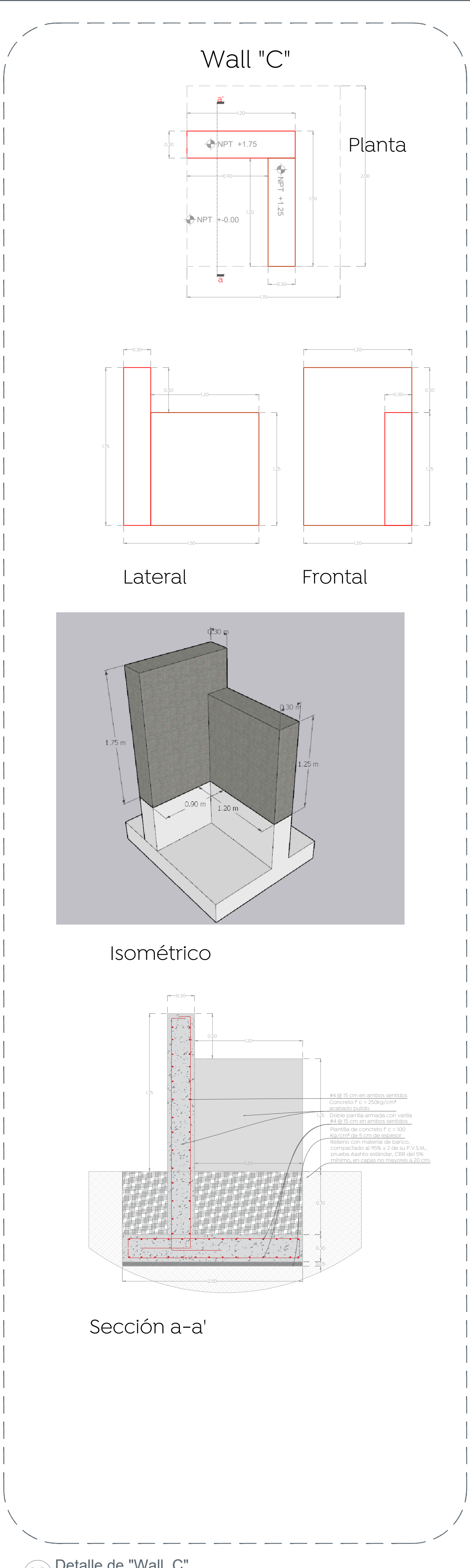
02 Detalle de "Wall C" PARKOUR 1:30
