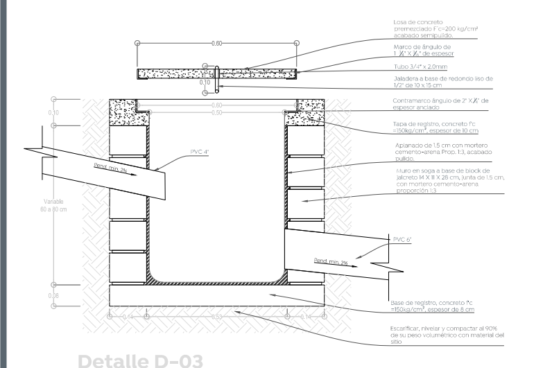
04 Detalle registro D-03 S/E
