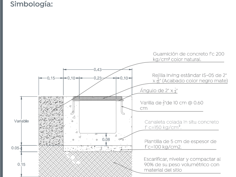
03 Detalle rejilla D-02 S/E
