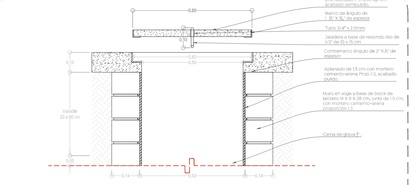
04 Detalle registro D-01 S/E
