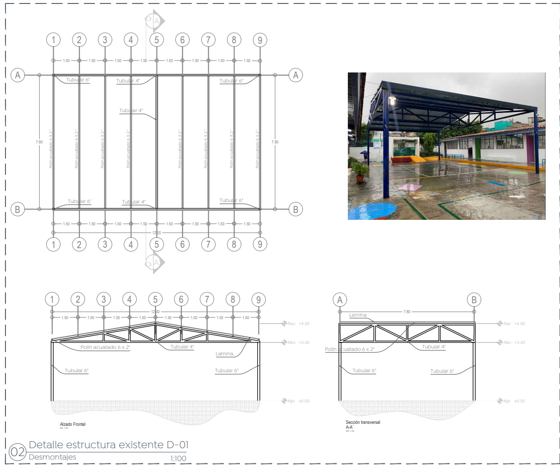
02 Detalle estructura existente D-01 Desmontajes 1:100
