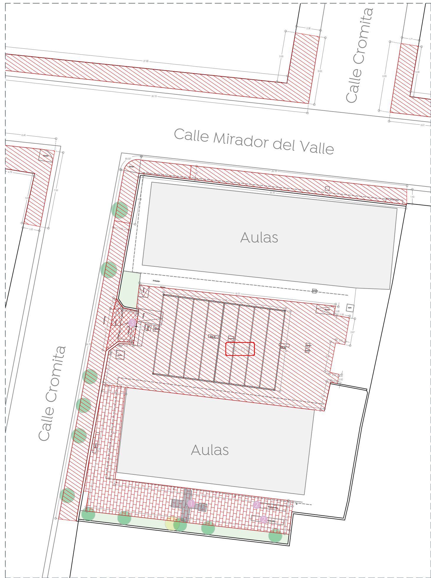
01 Planta de Conjunto Demoliciones | Estado actual 1:100
