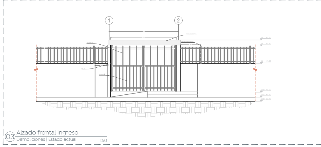
03 Alzado frontal ingreso Demoliciones | Estado actual 1:50
