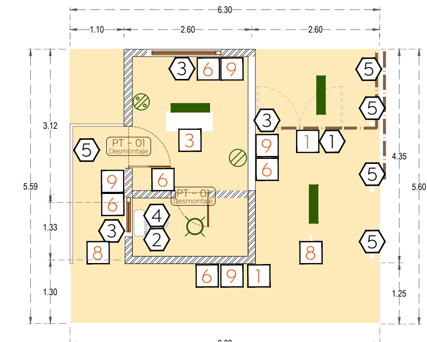
DM-Caseta Planta baja caseta CEMAM Esc. 1:75
