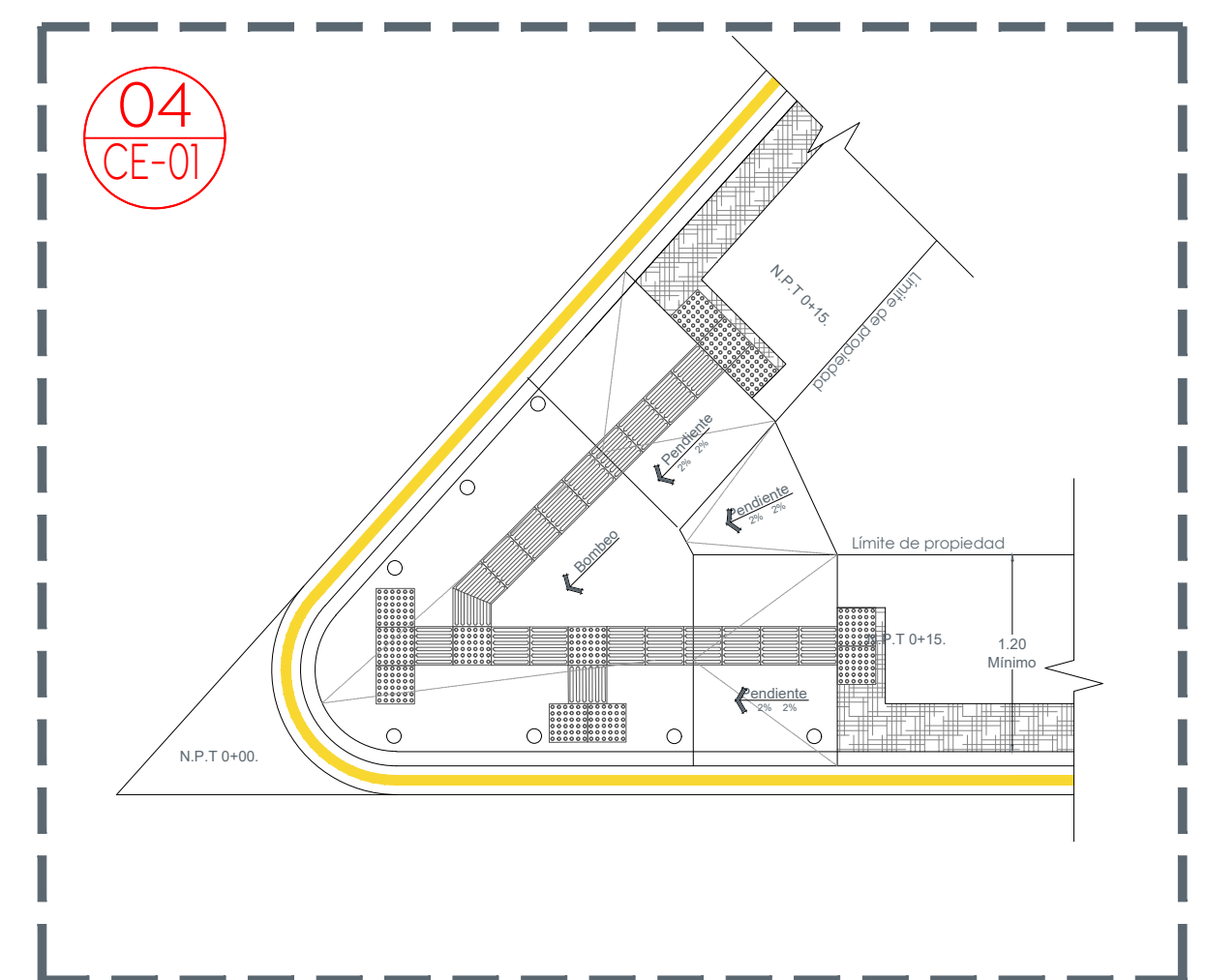
04 Detalle de esquina ángulo agudo Validar aplicación según proyecto
