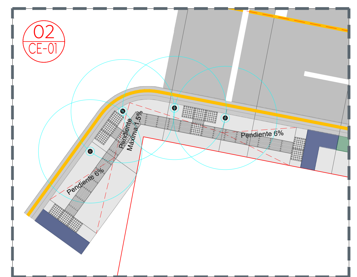
02 Detalle de esquina ángulo agudo Validar aplicación según proyecto
