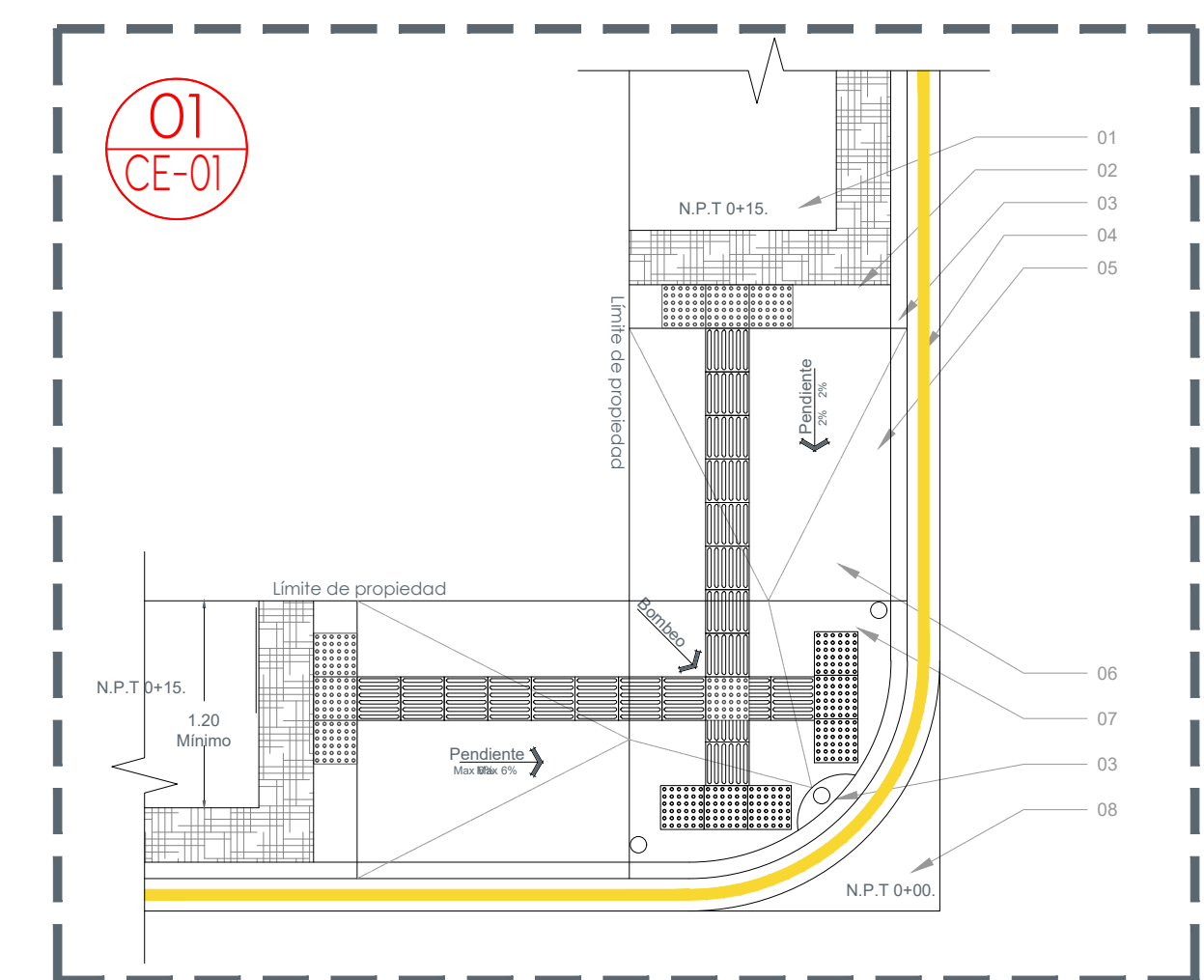
01 Esquina común Validar aplicación según proyecto
