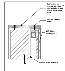
DETALLE - JAMBA DE MADERA ESC. 1:1
