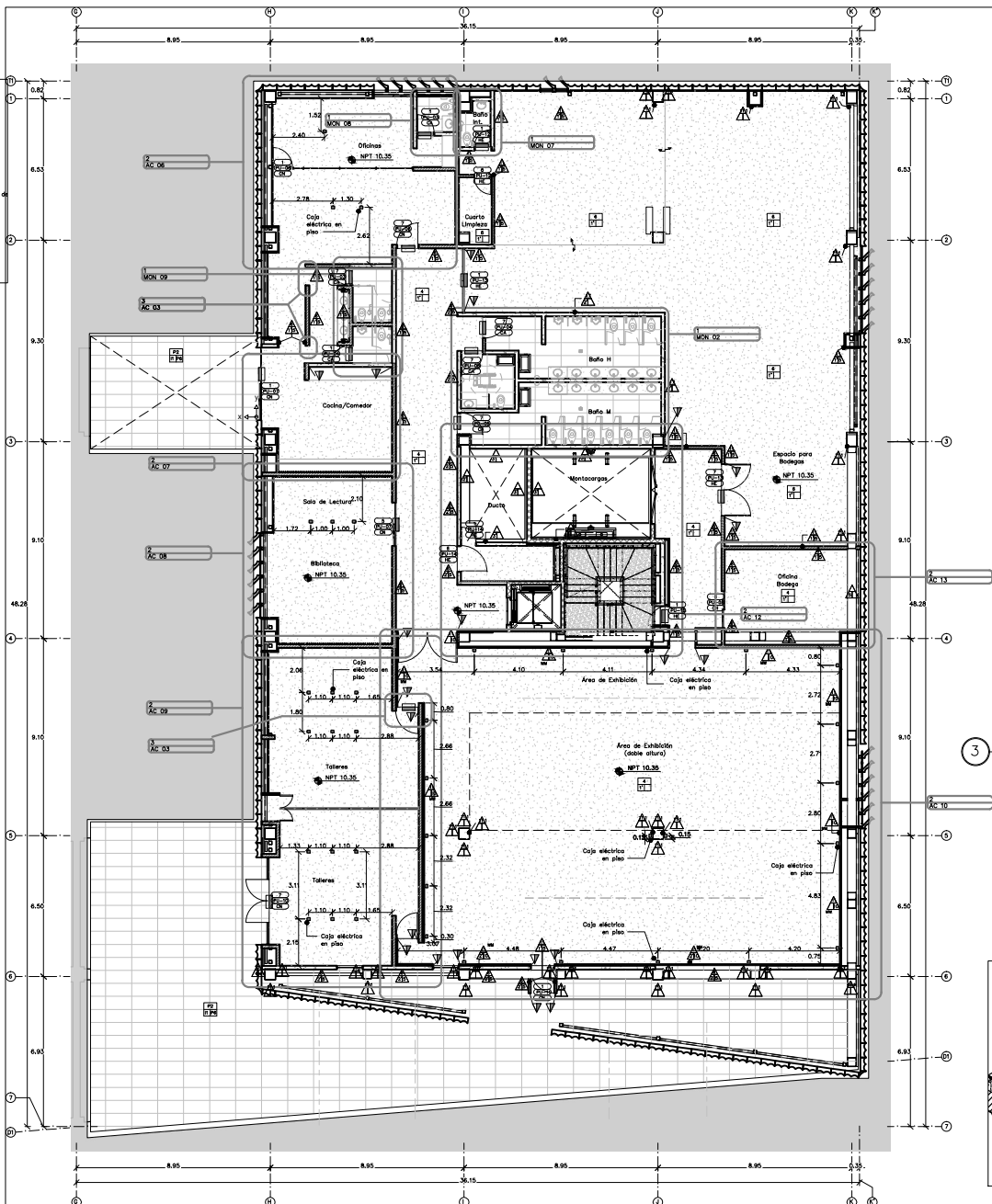
NIVEL 2 ACABADOS ESC. 1:100
