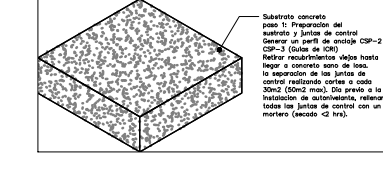
DETALLE PISO AUTONIVELANTE ESC. 1:20
