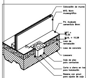
DETALLE TIPO - CAJA ELÉCTRICA EN PISO ESC. 1:1
