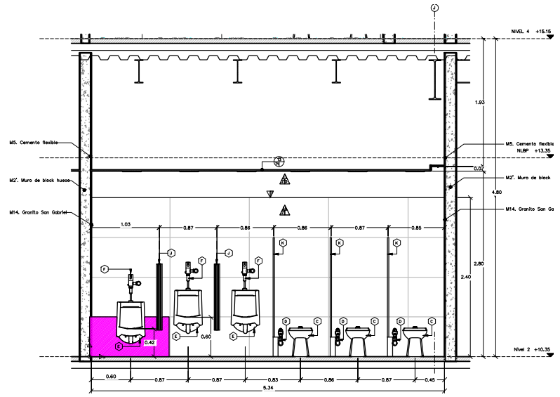
1 SECCIÓN 3 BAÑOS H./M. - NIVEL 2 ESC. 1:1
