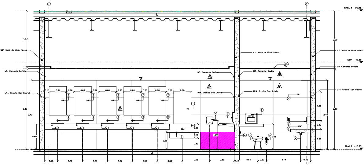
2 SECCIÓN 4 BAÑOS H./M. - NIVEL 2 ESC. 1:1
