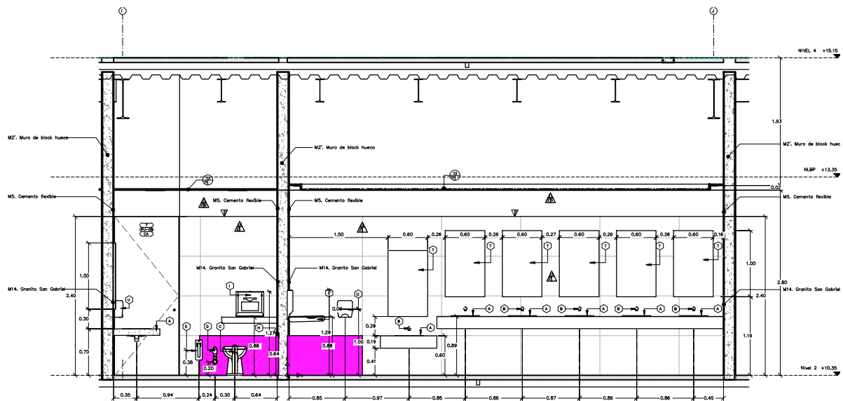
3 SECCIÓN 5 BAÑOS H./M. - NIVEL 2 ESC. 1 : 25
