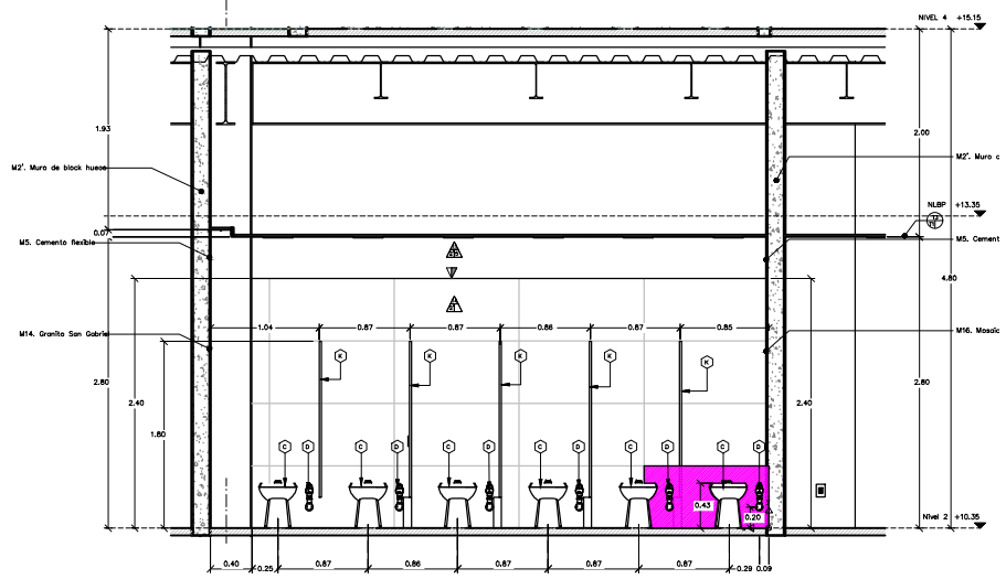
2 SECCIÓN 6 BAÑOS H./M. ESC. 1 : 25
