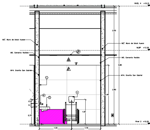
2 SECCIÓN 8 BAÑO DISCAPACITADOS – NIVEL 2 ESC. 1 : 25
