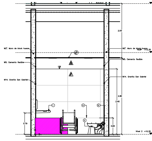
1 SECCIÓN 7 BAÑO DISCAPACITADOS – NIVEL 2 ESC. 1 : 25
