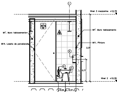
4 SECCIÓN 2 BAÑO BODEGA ESC. 1 : 25
