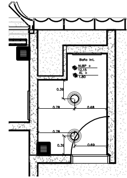
2 BAÑO BODEGA – PLAFONES ESC. 1 : 25
