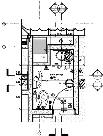
1 BAÑO BODEGA – NIVEL 2 ESC. 1 : 25
