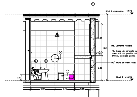
6 SECCIÓN 4 BAÑO BODEGA ESC. 1 : 25
