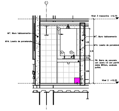
3 SECCIÓN 1 BAÑO BODEGA ESC. 1 : 25
