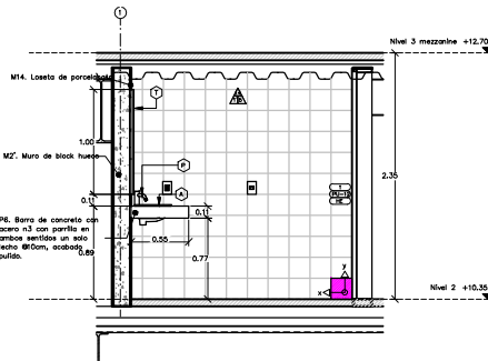
5 SECCIÓN 3 BAÑO BODEGA ESC. 1 : 25
