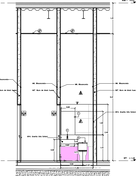
3 SECCIÓN 1 BAÑO ESC. 1 : 25
