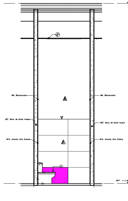
4 SECCIÓN 2 BAÑO ESC. 1 : 25
