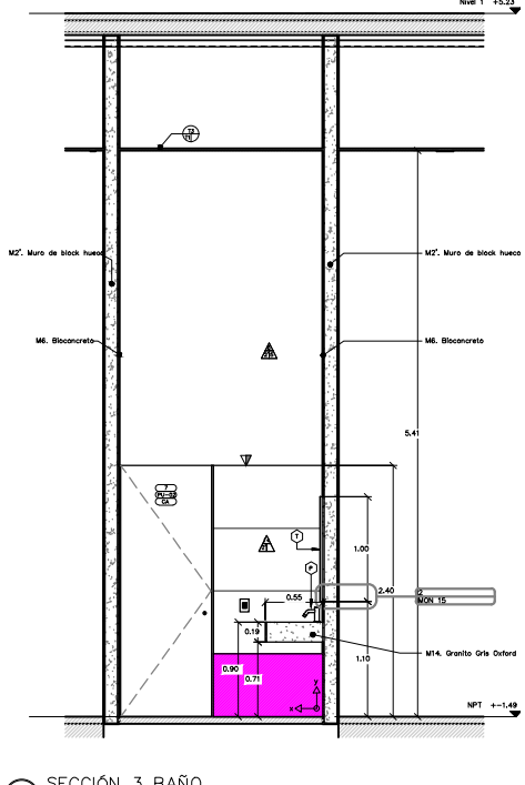
5 SECCIÓN 3 BAÑO ESC. 1 : 25
