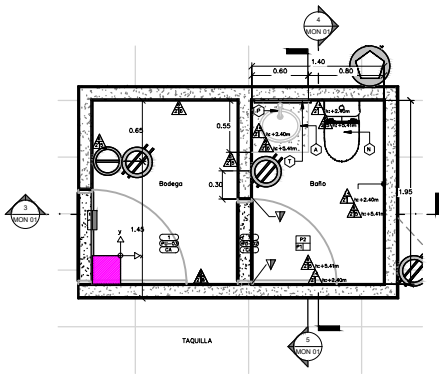
1 BAÑO – PLANTA BAJA ESC. 1 : 25
