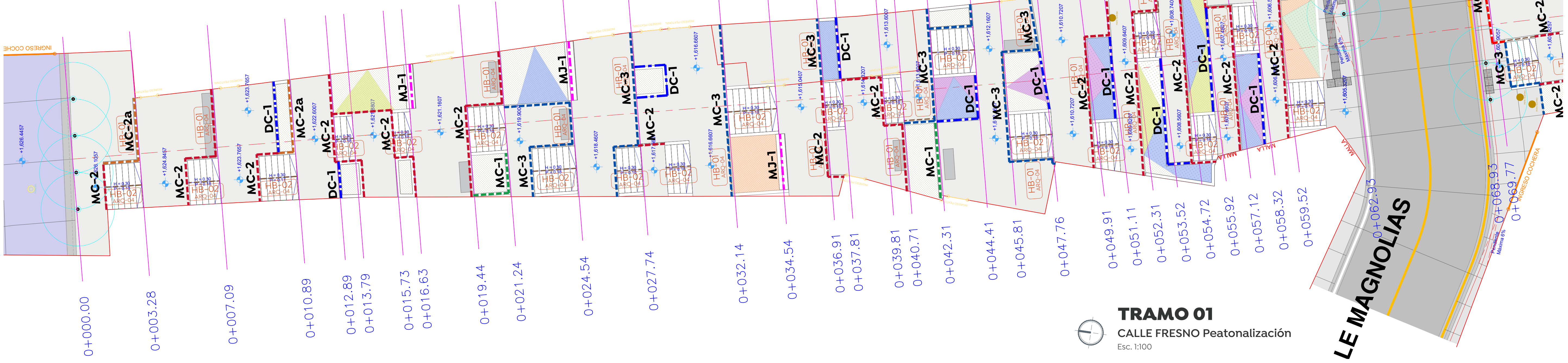
Planta general Escala 1:500
