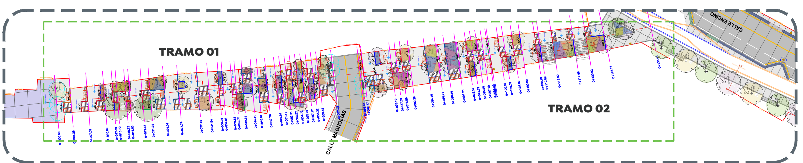
Planta general Escala 1:500
