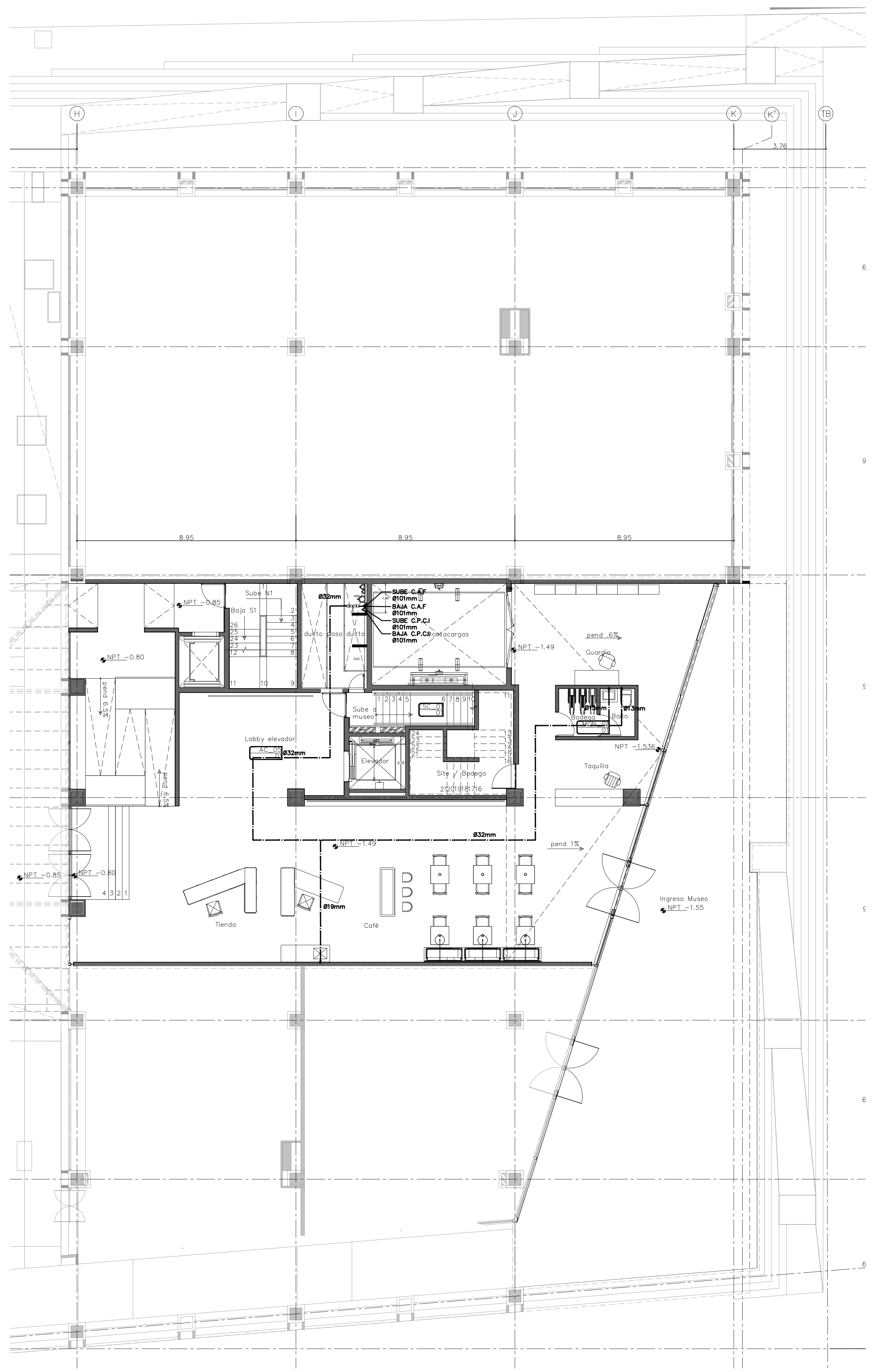
01 PLANTA BAJA 1:100
