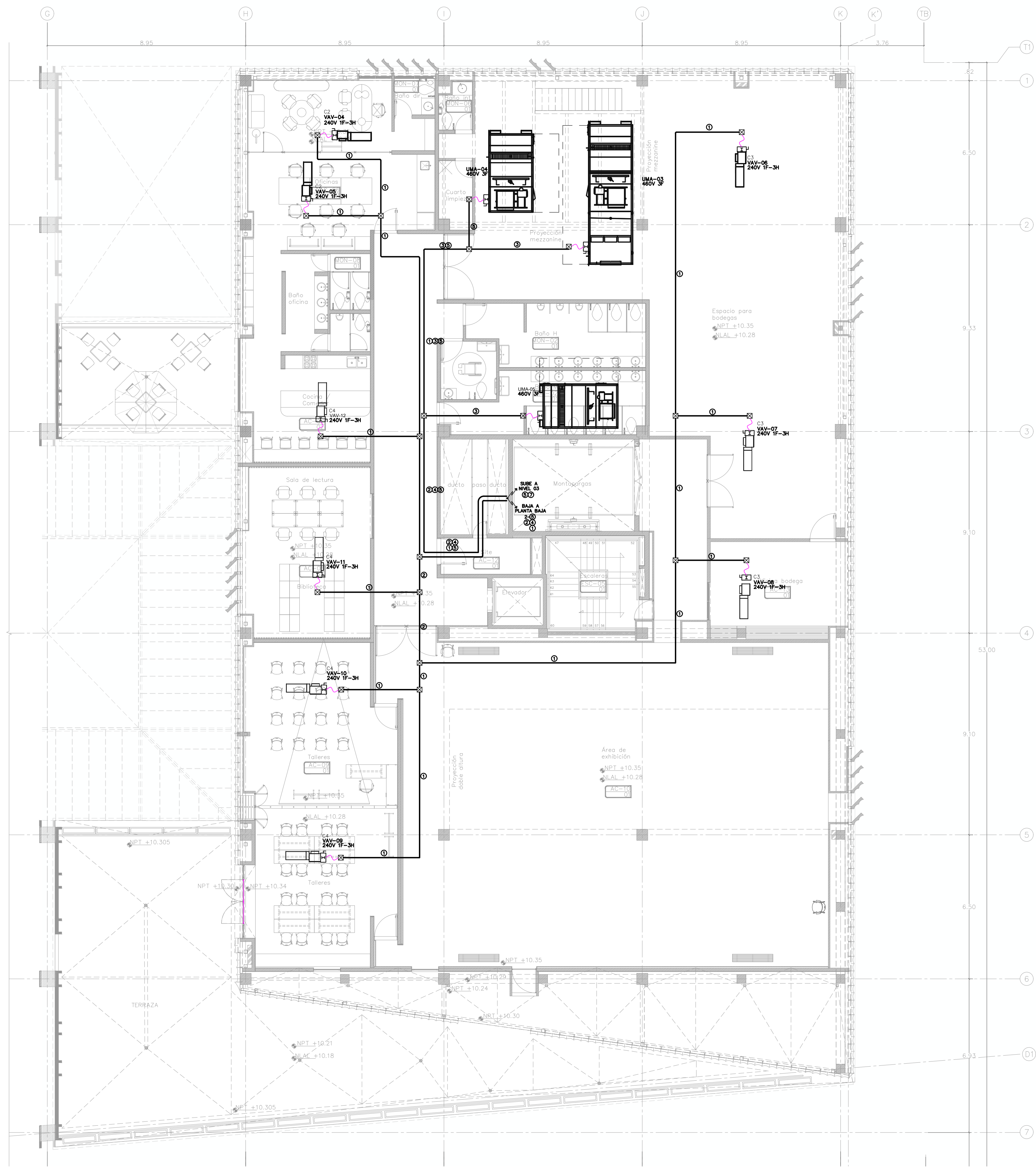
INSTALACION ELECTRICA, CONTACTOS NIVEL 02 ESC. 1:100
