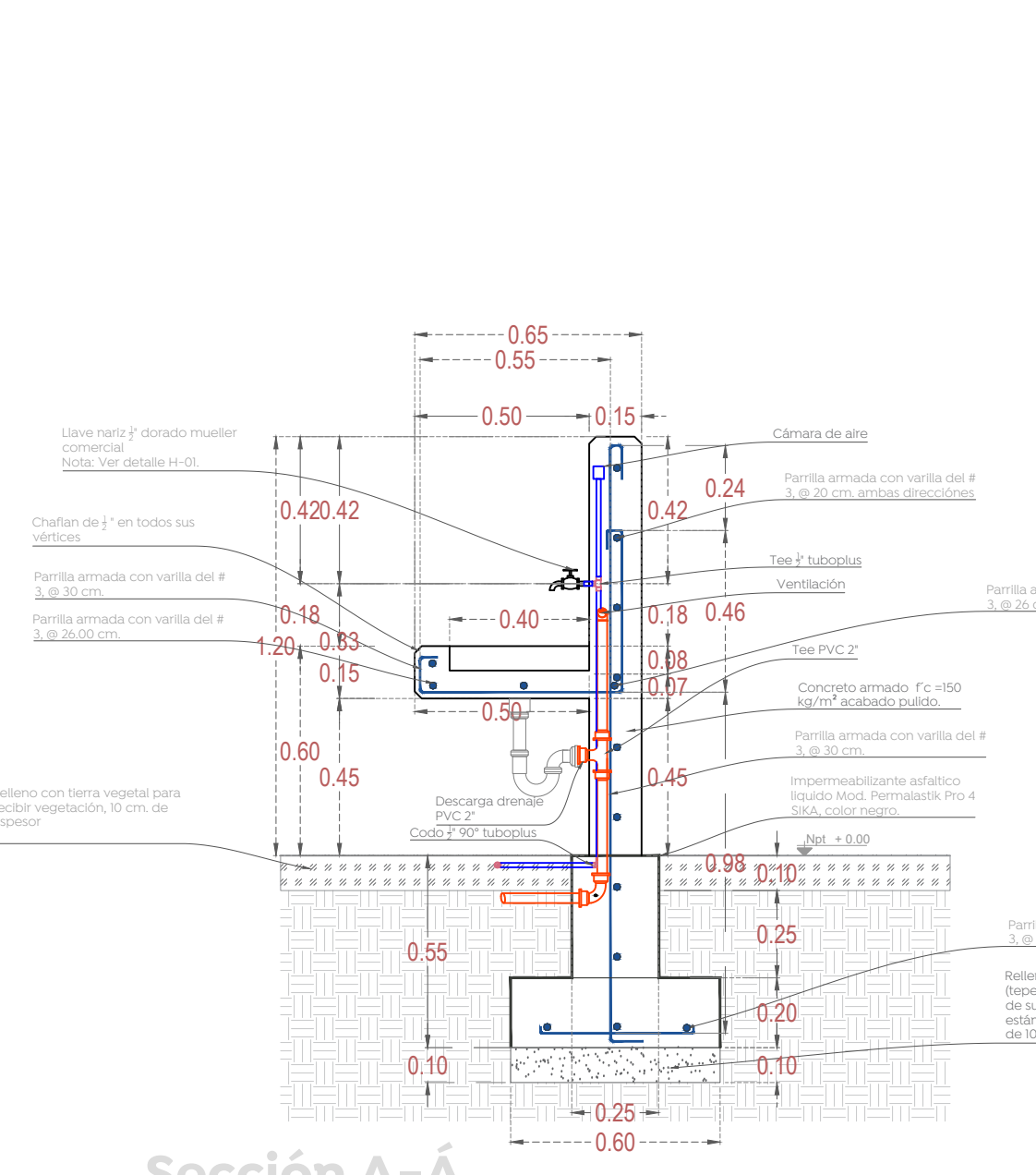
02 Detalle de lavamanos Detalle D-01 1:20
