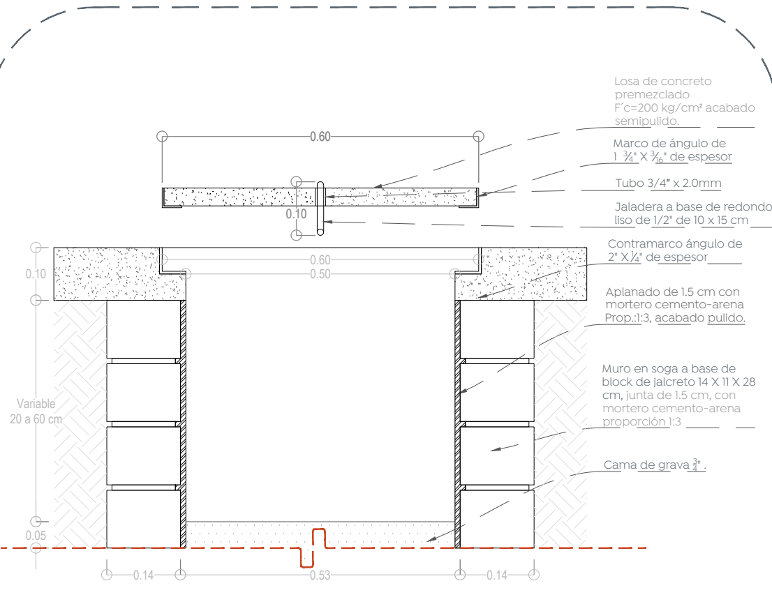
03 Detalle de registro Detalle D-01 1:10
