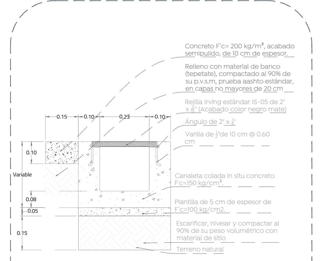
04 Detalle de rejilla Detalle D-02 1:10
