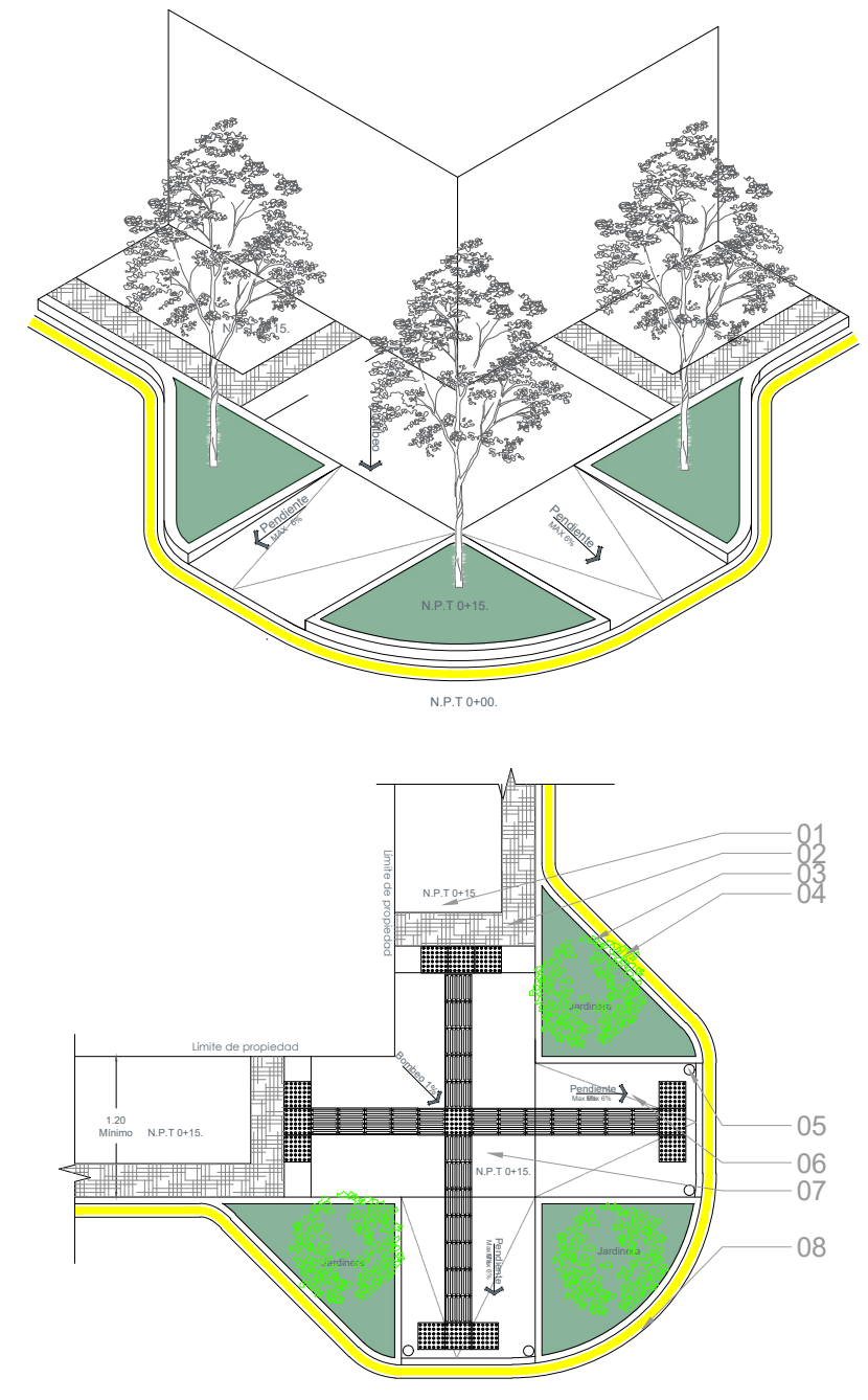
1.1 Esquinas Tipo, oreja doble
