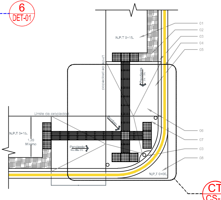
1 Detalle de esquina Esc. 1:10
