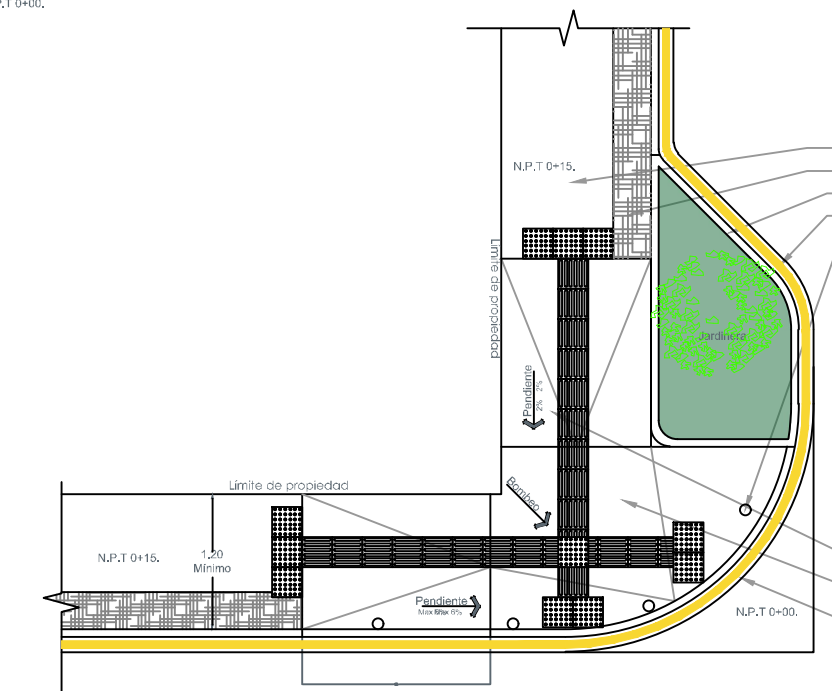
2 Detalle de esquina con bahía Esc. 1:10
