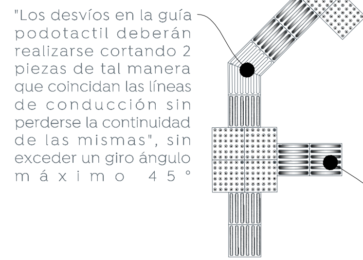
Figura No. 2.1.d. Cambios de dirección.
