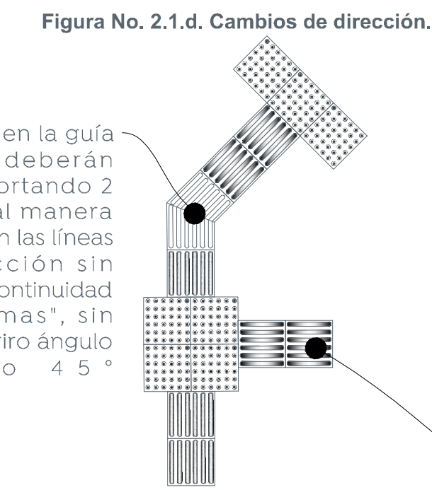
Figura No. 2.1.d. Cambios de dirección.
