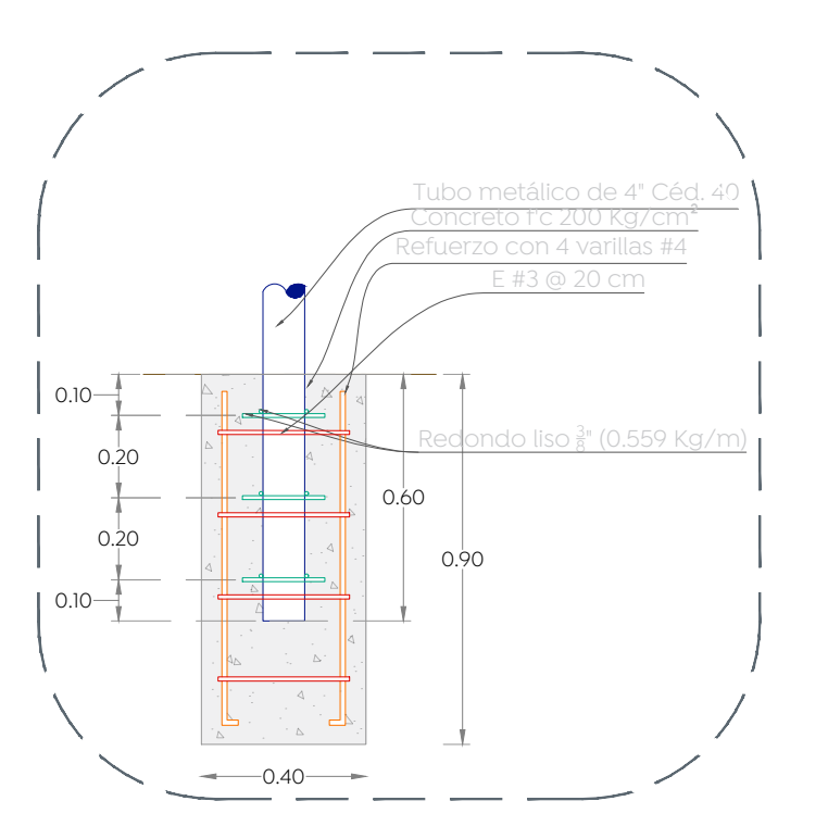
06 Dado de tablero d.3 1:20
