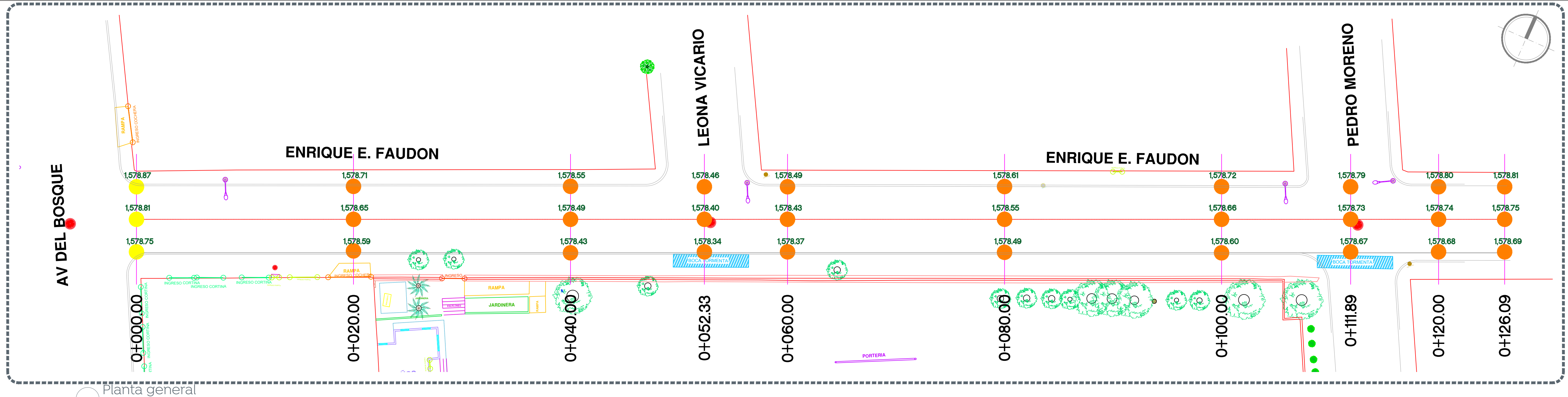
Planta general Escala 1:3000
