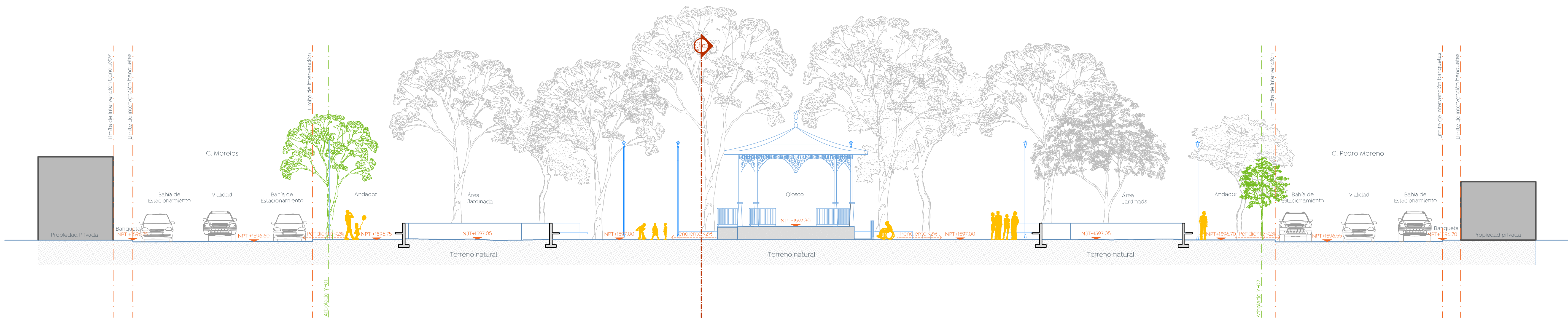
01 Sección Longitudinal A-A' Estado Propuesto 1:125
