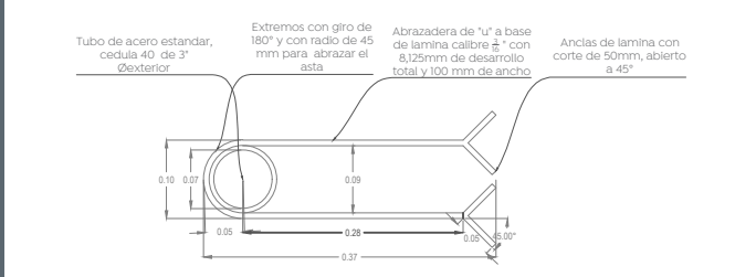
Detalle A-02
