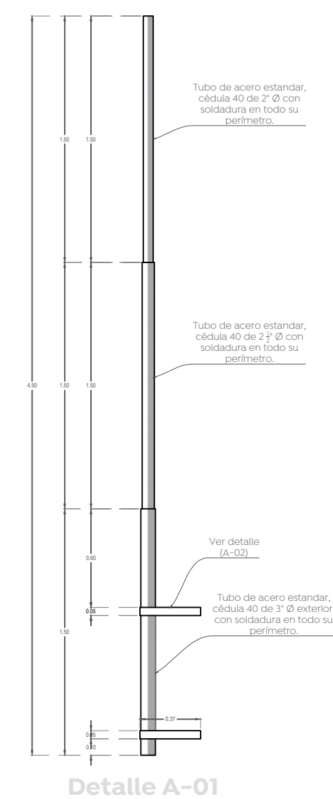
Detalle A-01
