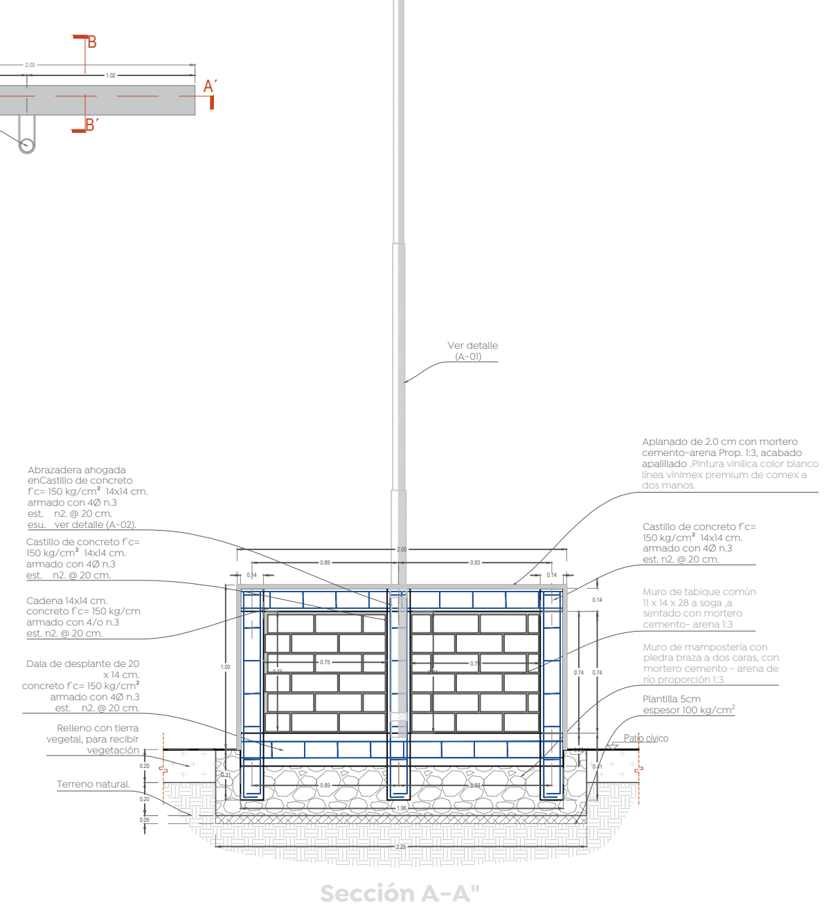
Sección A-A
