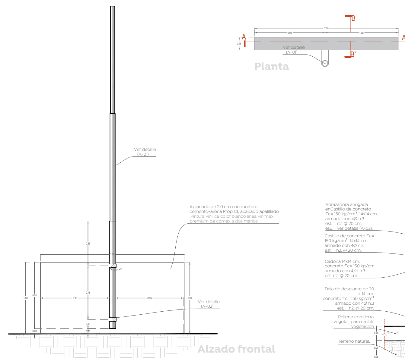
Alzado frontal
