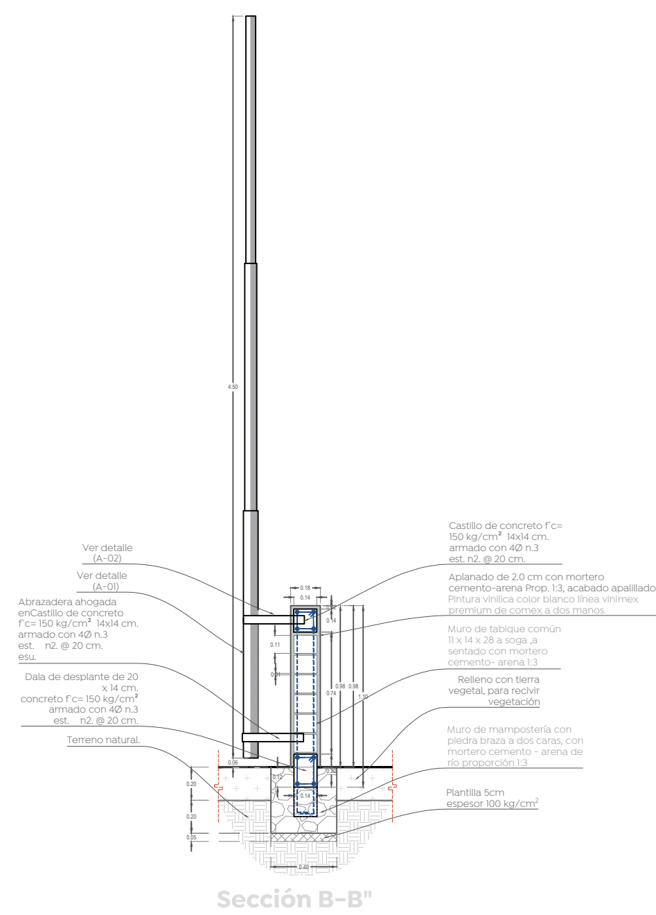
Sección B-B
